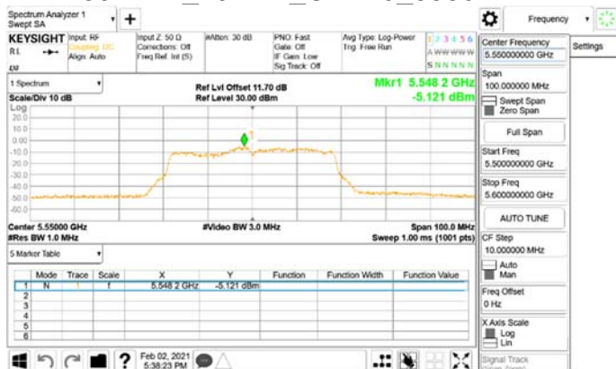
802.11n_40MHz_Chain0_5550MHz
