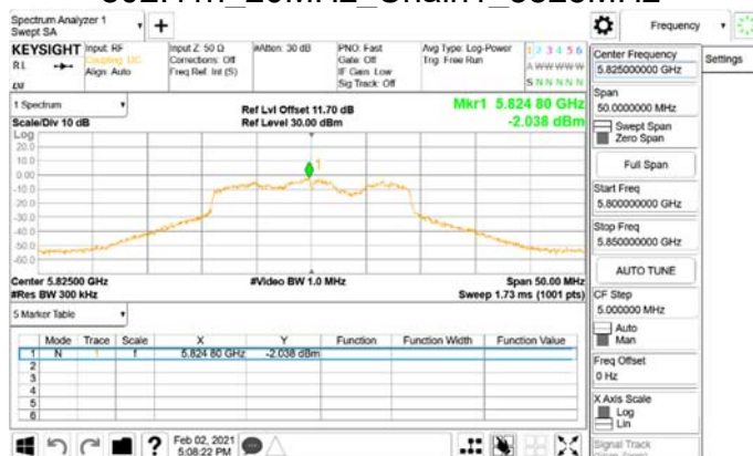
802.11n_20MHz_Chain1_5825MHz
