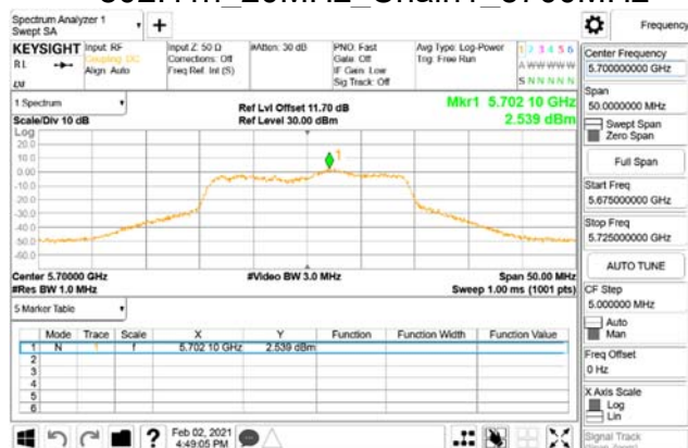
802.11n_20MHz_Chain1_5700MHz
