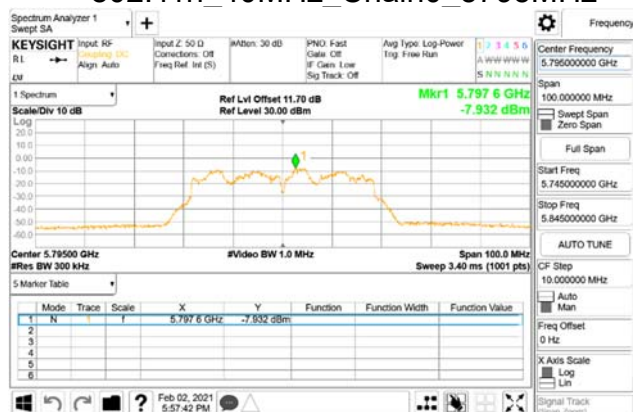
802.11n_40MHz_Chain0_5795MHz
