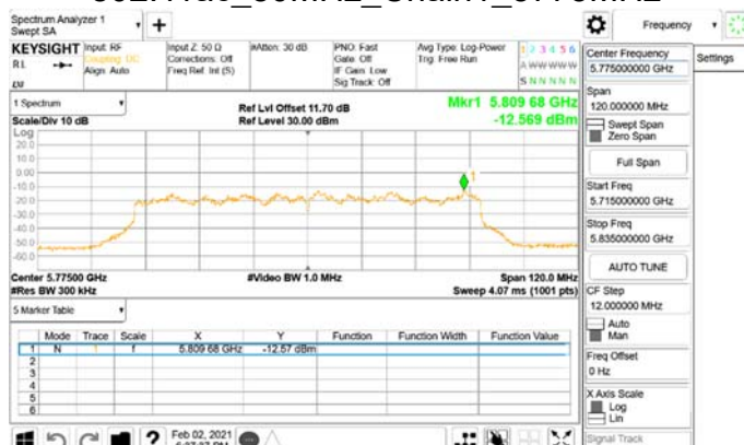
802.11ac_80MHz_Chain1_5775MHz
