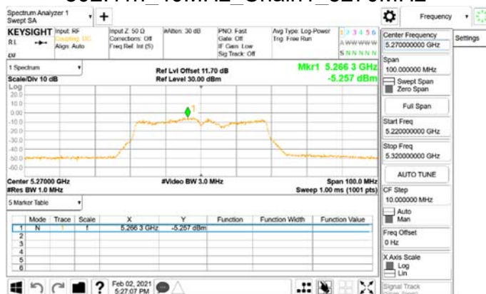
802.11n_40MHz_Chain1_5270MHz
