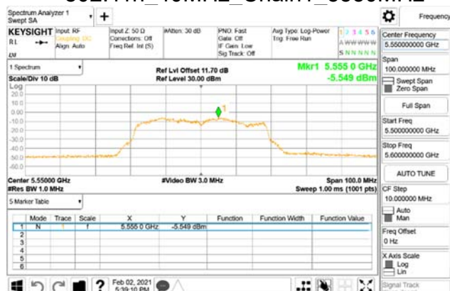
802.11n_40MHz_Chain1_5550MHz
