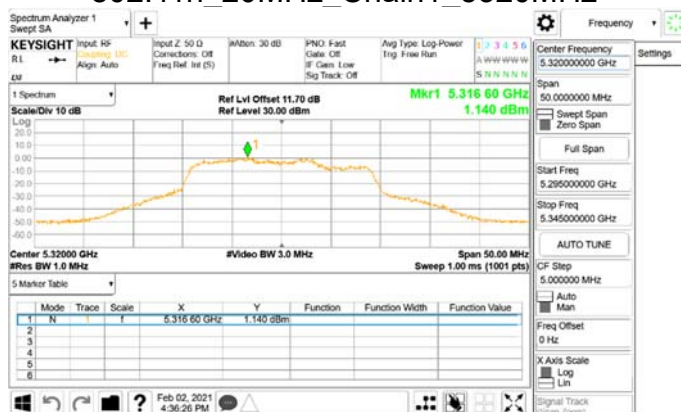
802.11n_20MHz_Chain1_5320MHz
