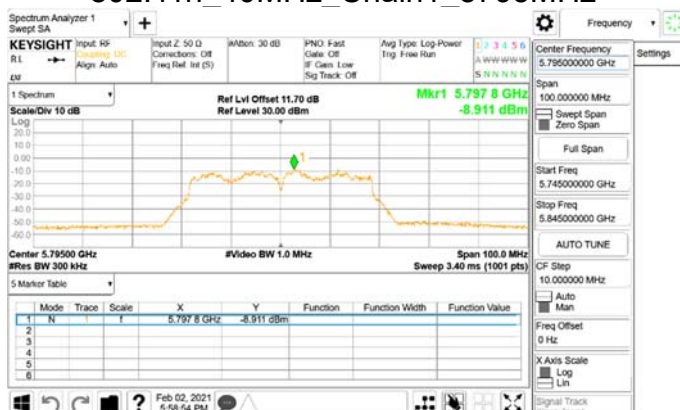
802.11n_40MHz_Chain1_5795MHz
