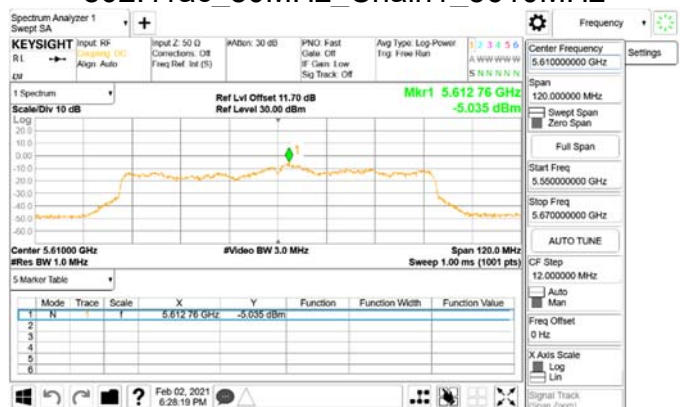
802.11ac_80MHz_Chain1_5610MHz
