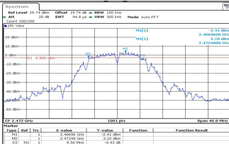
11B_Ant1_2472
