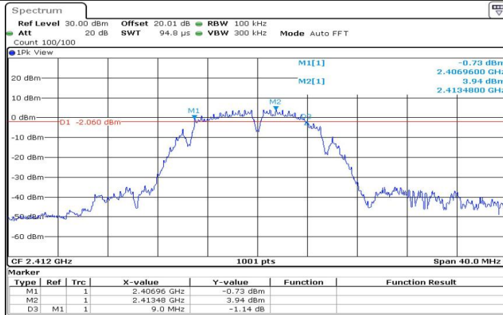
11B_Ant1_2412
