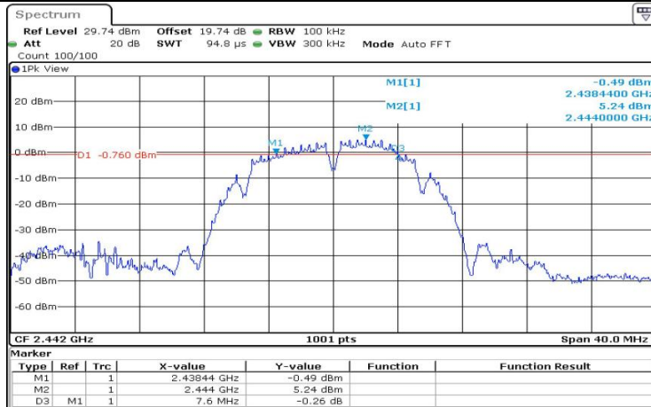
11B_Ant1_2442
