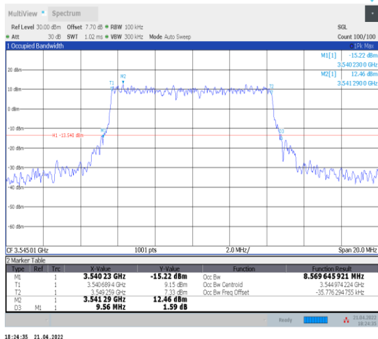
1-N78-3450-3550--30-10-H-3-DFT-16QAM-Outer_Fu ll-24@0-Ant0-8.57-9.560-≤10-PASS
