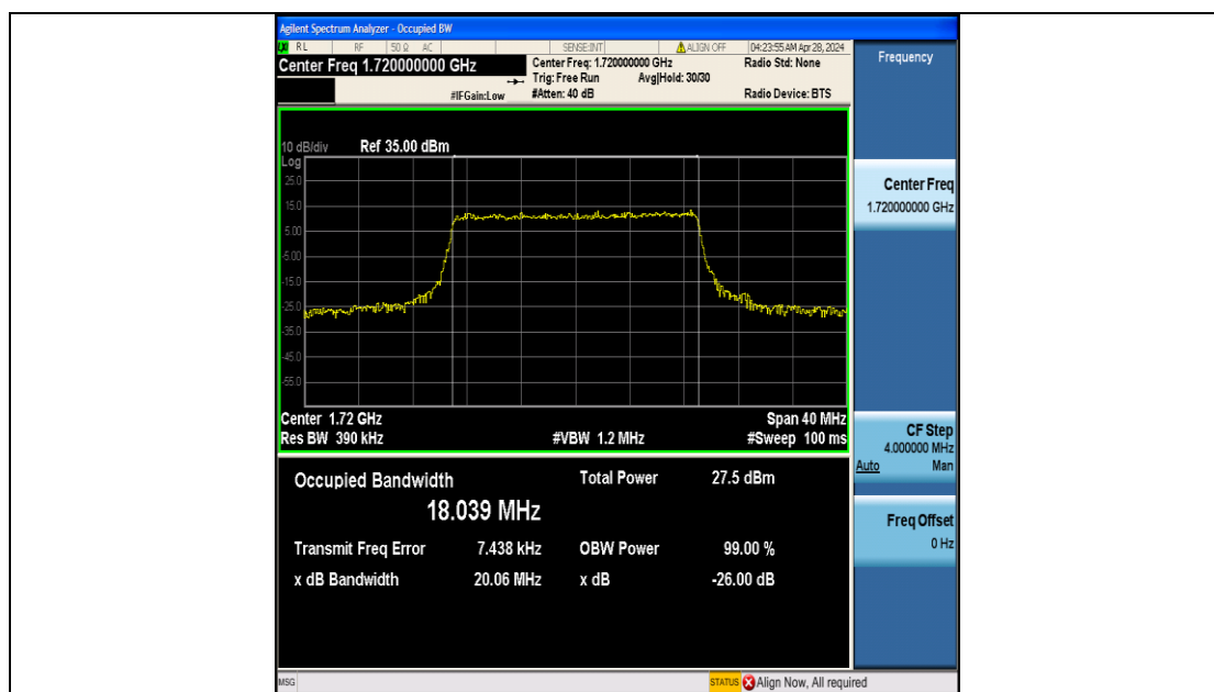
Band4-20MHz-QPSK-20050-100RB#0-PASS
