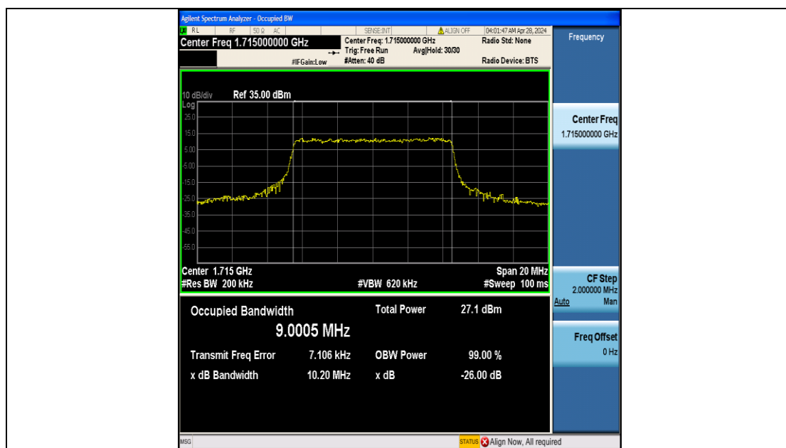
Band4-10MHz-QPSK-20000-50RB#0-PASS
