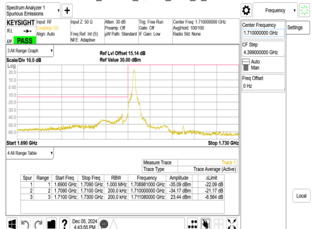
Band66_20MHz_QPSK_RB1_0_CH132072
