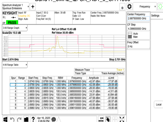
Band41_5MHz_QPSK_RB1_24_CH41565
