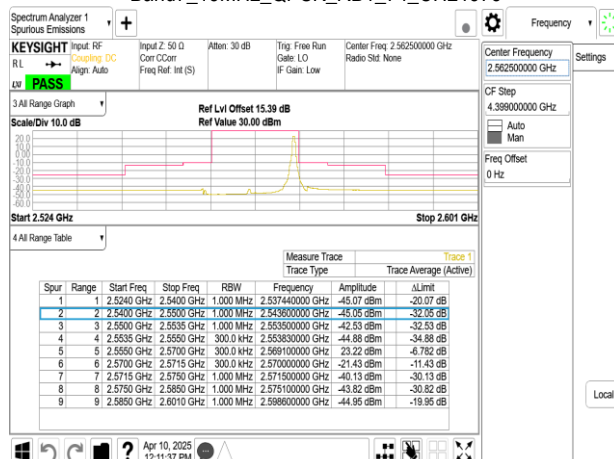
Band7_15MHz_QPSK_RB1_74_CH21375
