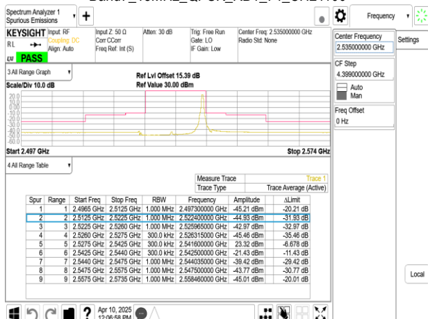
Band7_15MHz_QPSK_RB1_74_CH21100
