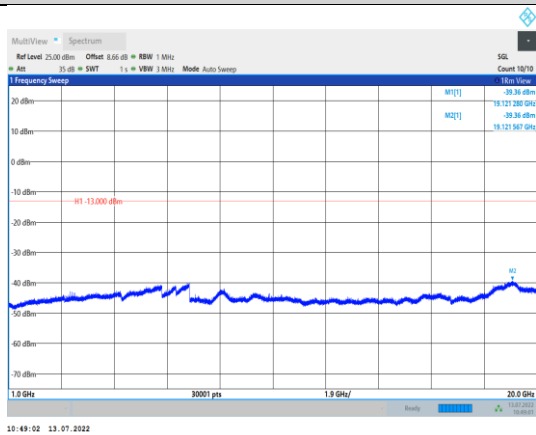
EGPRS1900-512-2-1000~20000MHz
