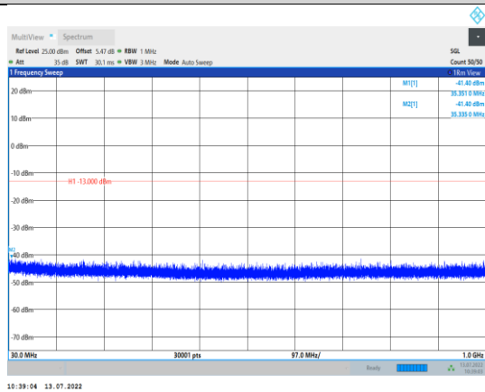
EGPRS850-190-8-30~1000MHz
