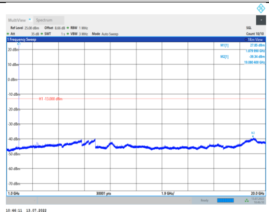
GSM1900-810-0-1000~20000MHz
