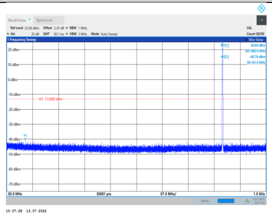
GPRS850-251-3-30~1000MHz
