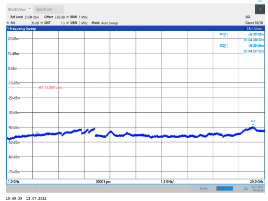
EGPRS1900-661-2-1000~20000MHz
