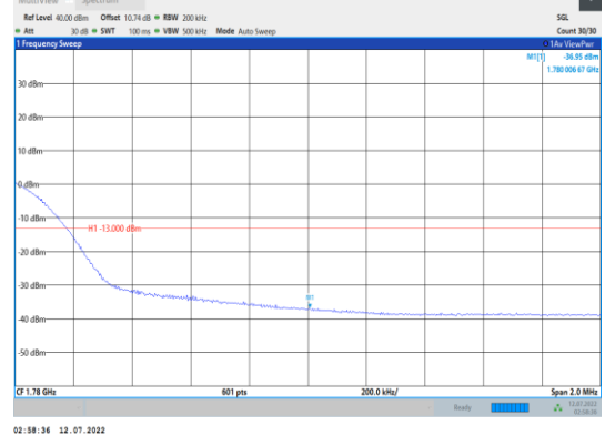
Band66-20MHz-QPSK-132572-100RB#0
