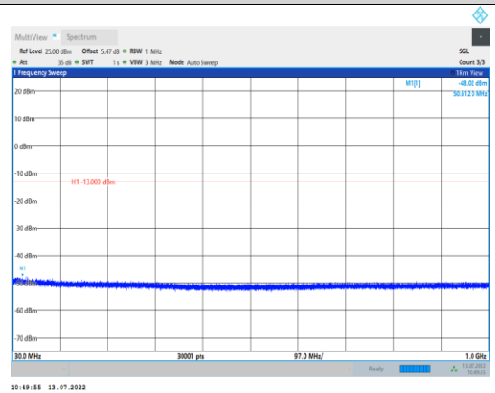
EGPRS1900-810-2-30~1000MHz
