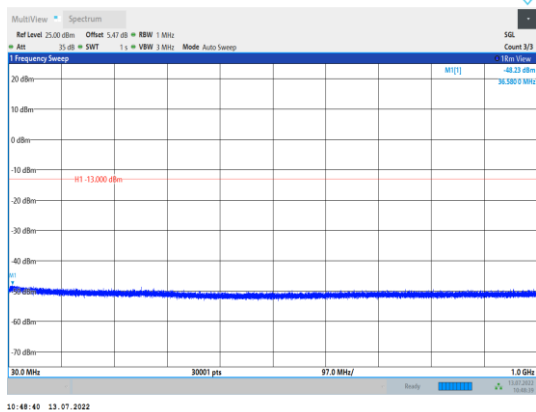
EGPRS1900-512-2-30~1000MHz
