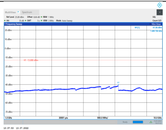
GPRS850-251-3-1000~10000MHz
