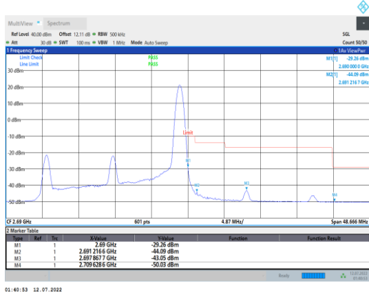
Band41-20MHz-16QAM-41490-1RB#99
