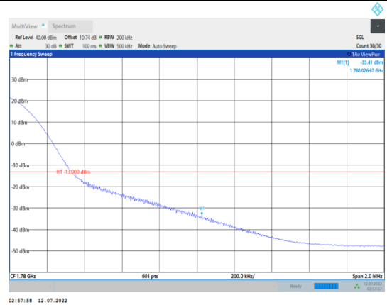
Band66-20MHz-QPSK-132572-1RB#99
