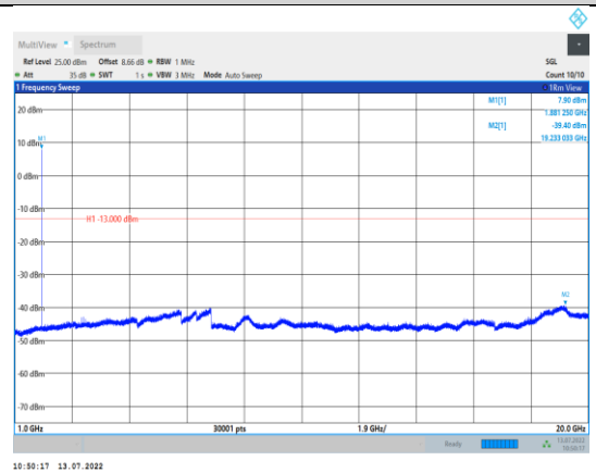
EGPRS1900-810-2-1000~20000MHz
