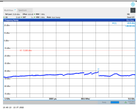
EGPRS850-251-8-1000~10000MHz
