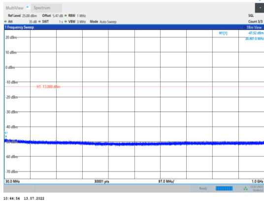
GSM1900-512-0-30~1000MHz
