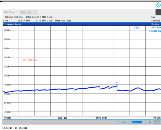
GPRS850-128-3-1000~10000MHz
