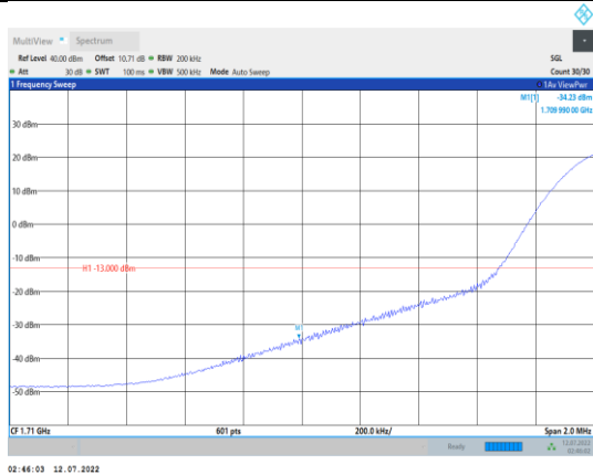
Band66-20MHz-QPSK-132072-1RB#0
