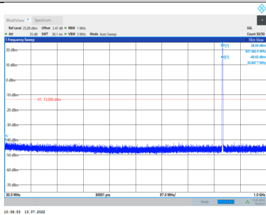
GPRS850-190-3-30~1000MHz
