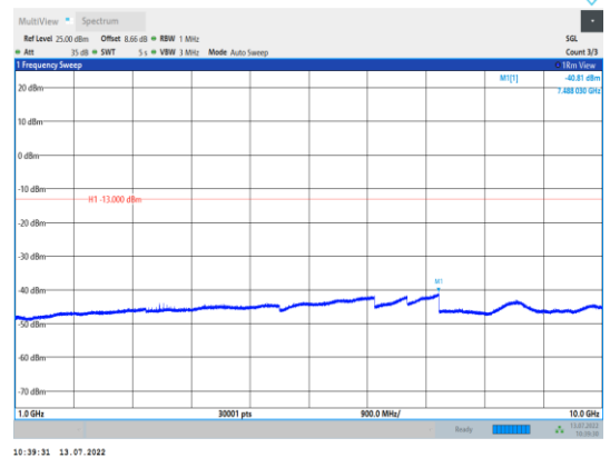
EGPRS850-190-8-1000~10000MHz
