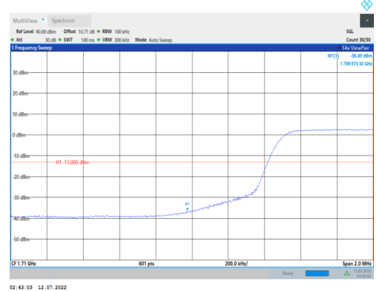
Band66-10MHz-QPSK-132022-50RB#0
