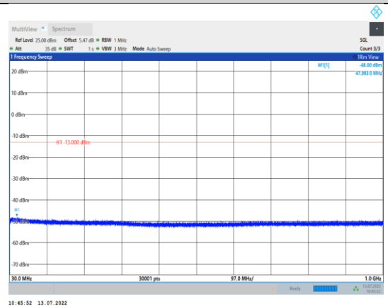
GSM1900-810-0-30~1000MHz
