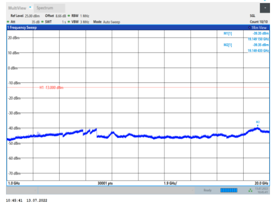
GSM1900-661-0-1000~20000MHz
