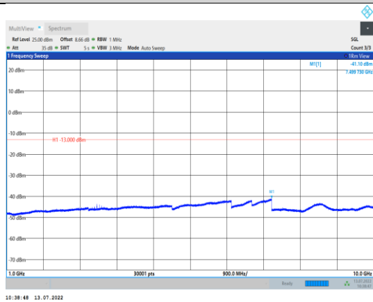
EGPRS850-128-8-1000~10000MHz
