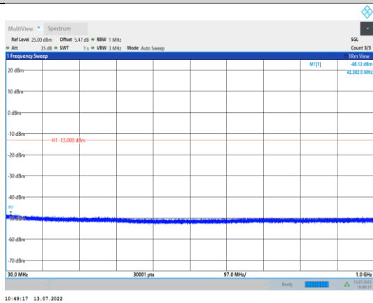
EGPRS1900-661-2-30~1000MHz
