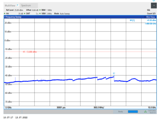
GPRS850-190-3-1000~10000MHz
