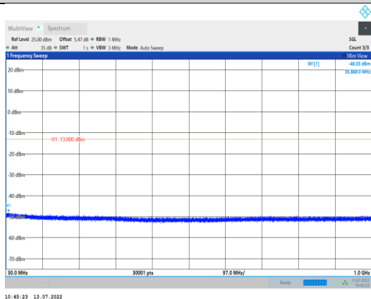
GSM1900-661-0-30~1000MHz
