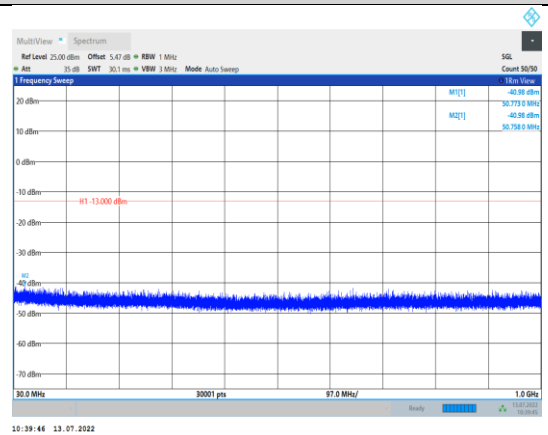
EGPRS850-251-8-30~1000MHz
