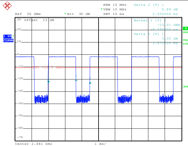
DH5_Ant1_2441
