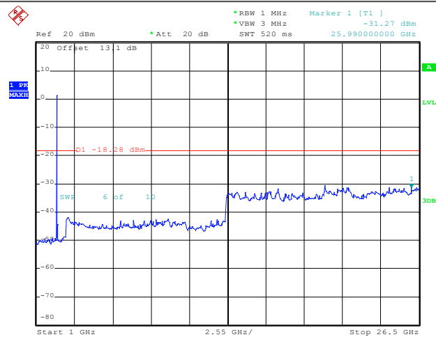
DH5_Ant1_2402_1000~26500
