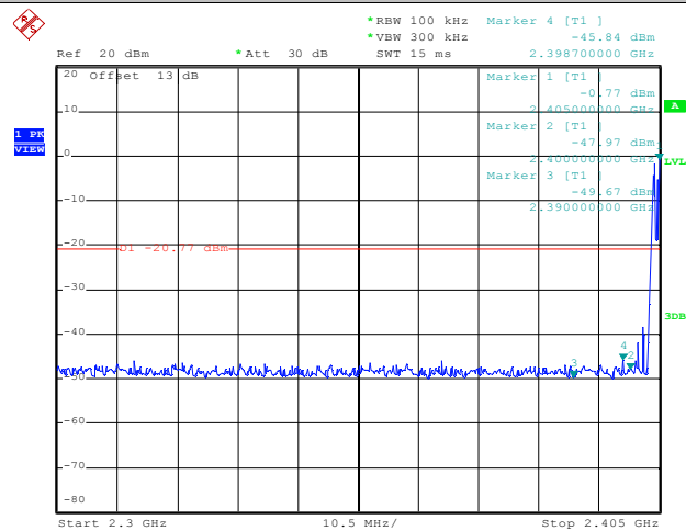
DH5_Ant1_Low_Hop_2402
