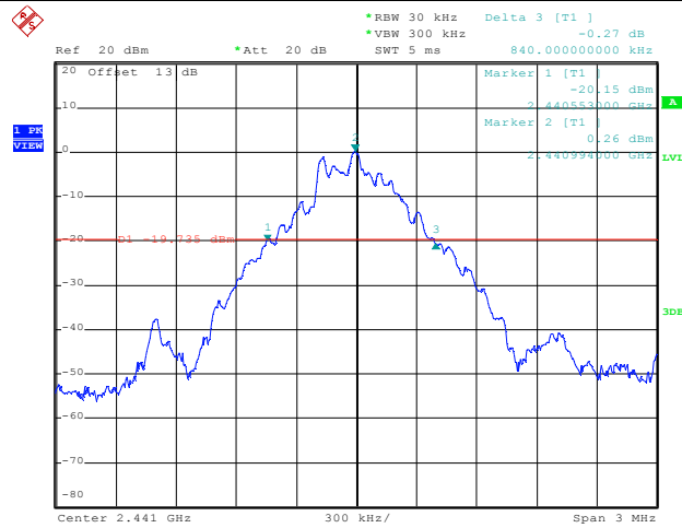
DH5_Ant1_2441
