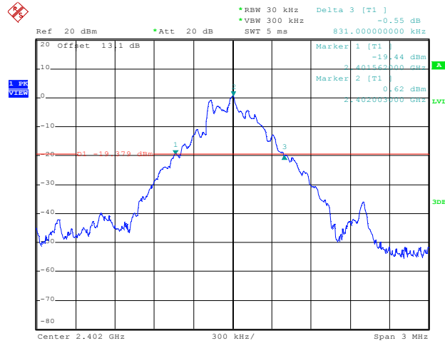
DH5_Ant1_2402
