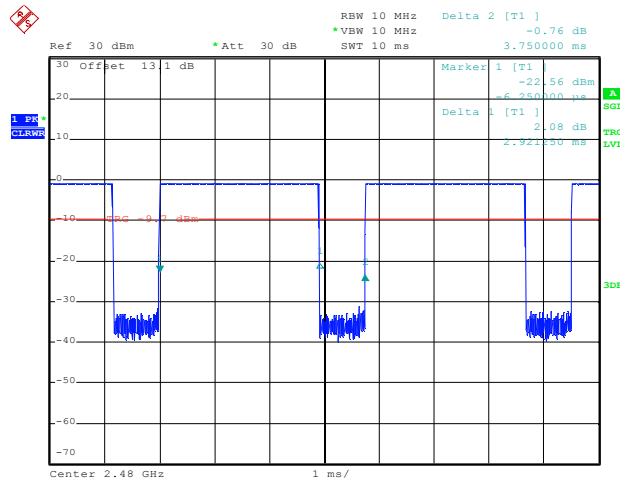
DH5_Ant1_2480
