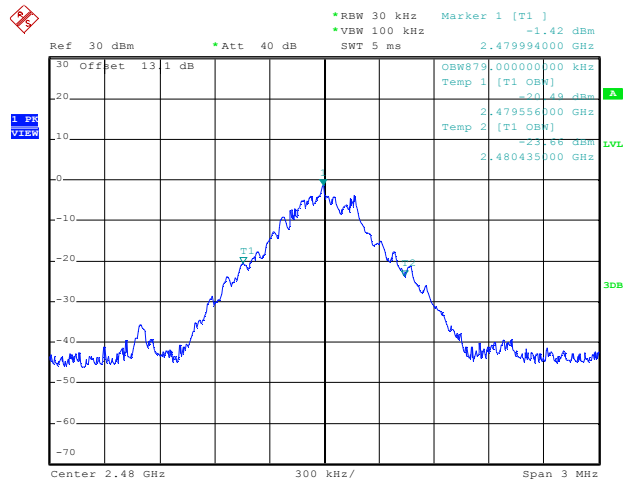
DH5_Ant1_2480
