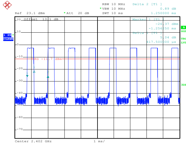
DH5_Ant1_2402
