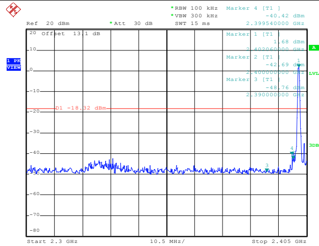
DH5_Ant1_Low_2402
