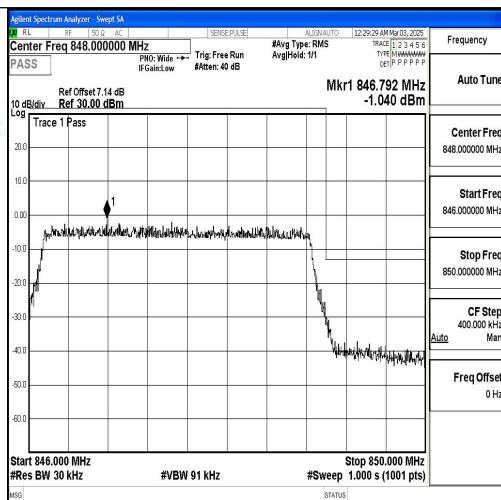
Band5_3MHz_16QAM_20635_15RB#0
