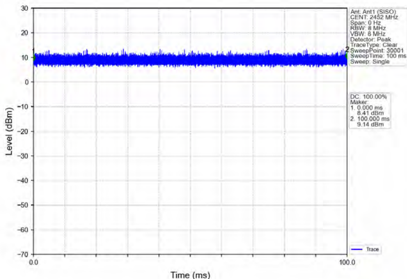
802.11n(HT40)_HCH_2452MHz_Ant1 (SISO)_NTNV
