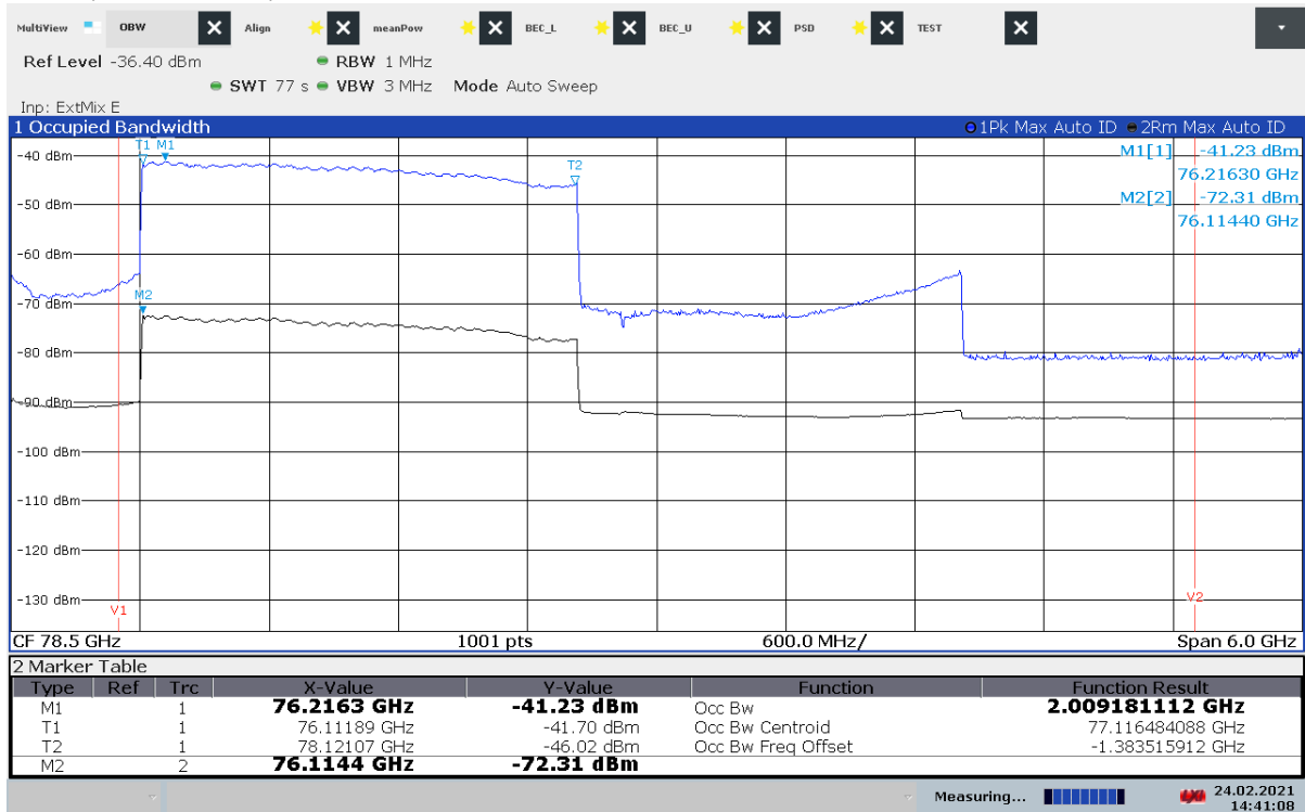
Plot 6: OBW, -30 °C / V nom , Mode 5
