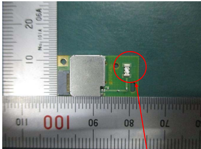
Antenna
