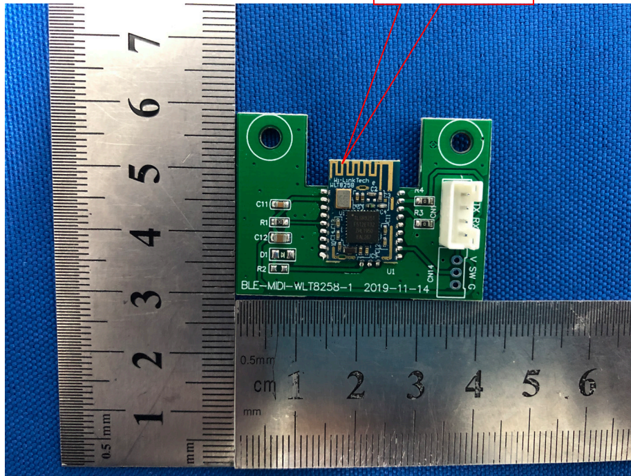
BLE Antenna
