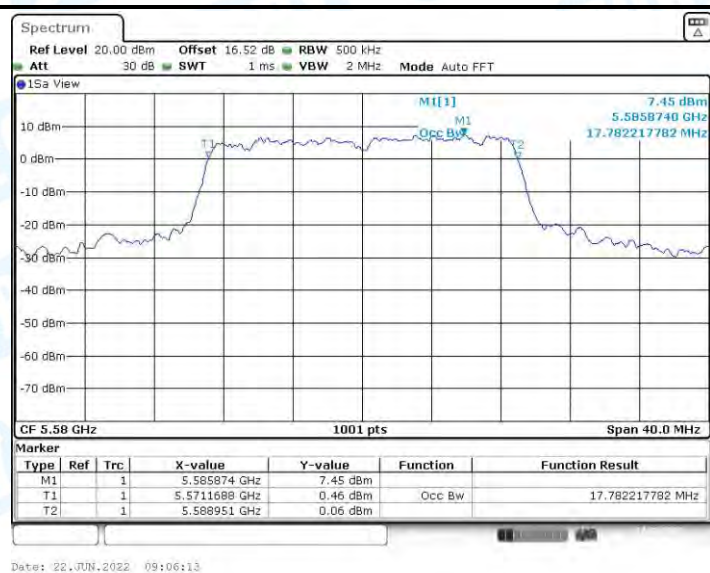
11N20MIMO_Ant2_5580
