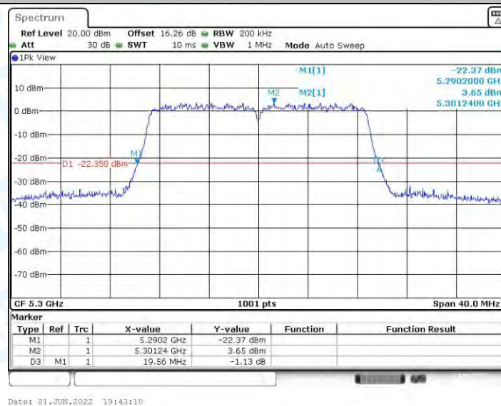
11N20MIMO_Ant1_5300
