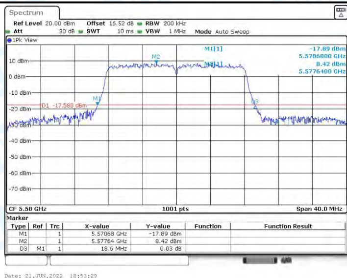
11A_Ant2_5580
