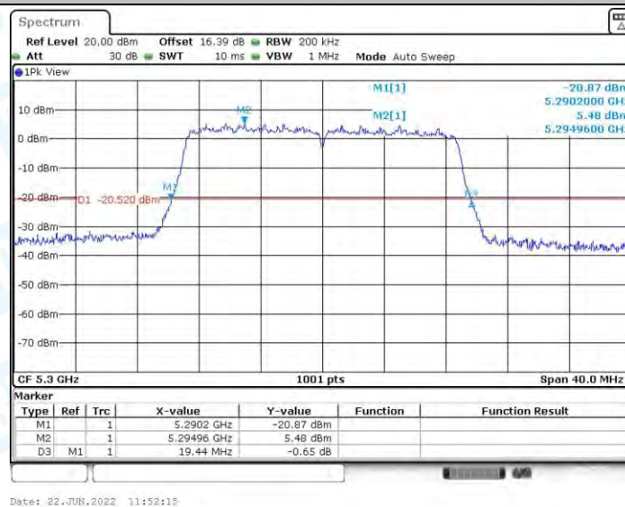
11AC20MIMO_Ant2_5300
