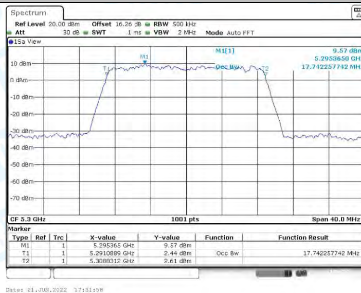
11A_Ant1_5300
