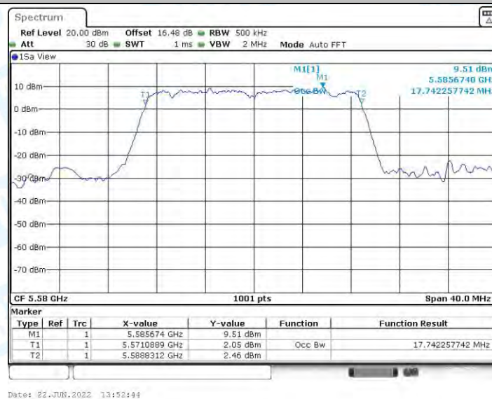
11AC20MIMO_Ant1_5580
