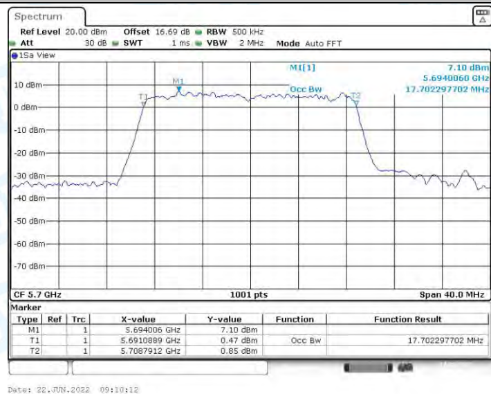
11N20MIMO_Ant1_5700
