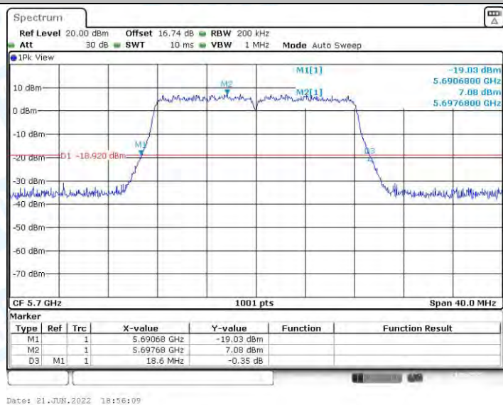
11A_Ant2_5700
