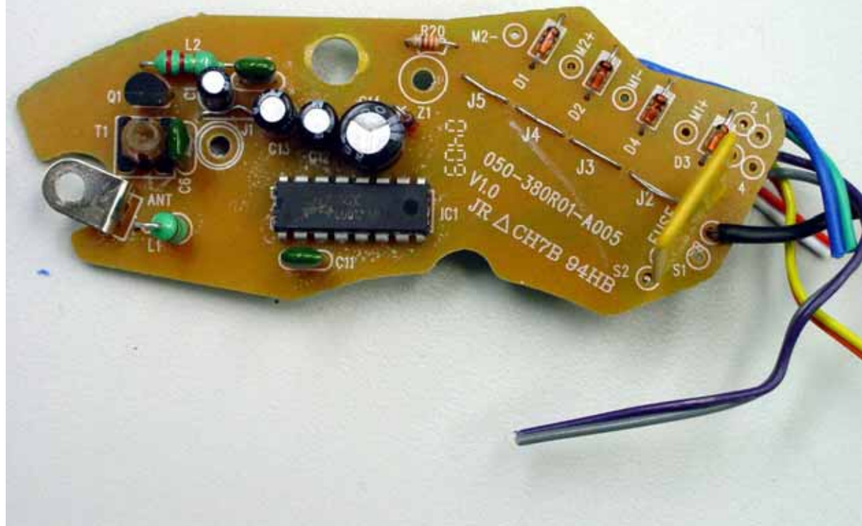
49MHz -RXPCB
