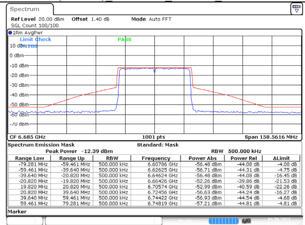
802.11ax (40MHz) 6685MHz Chain B NSS-1
