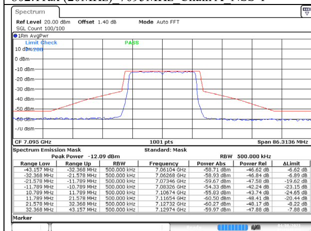
802.11ax (20MHz) 7095MHz Chain A NSS-1
