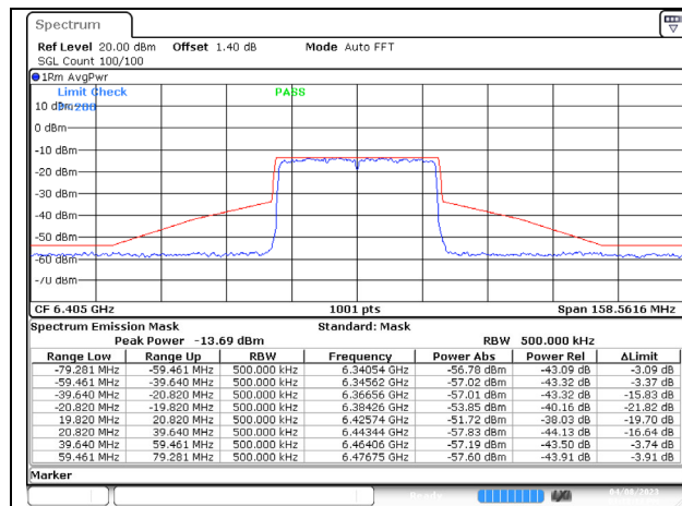
802.11ax (40MHz) 6405MHz Chain A NSS-1
