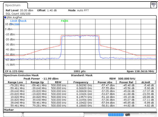
802.11ax (40MHz) 6125MHz Chain D NSS-1
