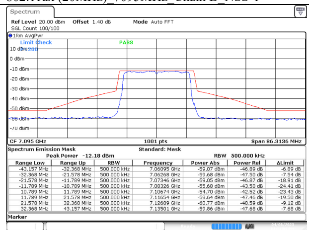
802.11ax (20MHz) 7095MHz Chain B NSS-1
