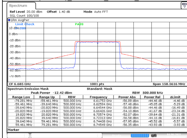
802.11ax (40MHz) 6685MHz Chain A NSS-1
