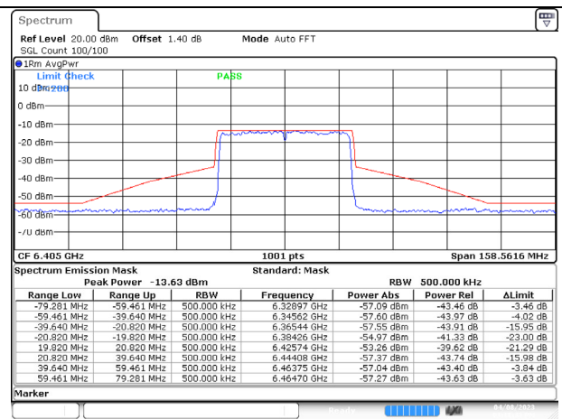
802.11ax (40MHz) 6405MHz Chain B NSS-1
