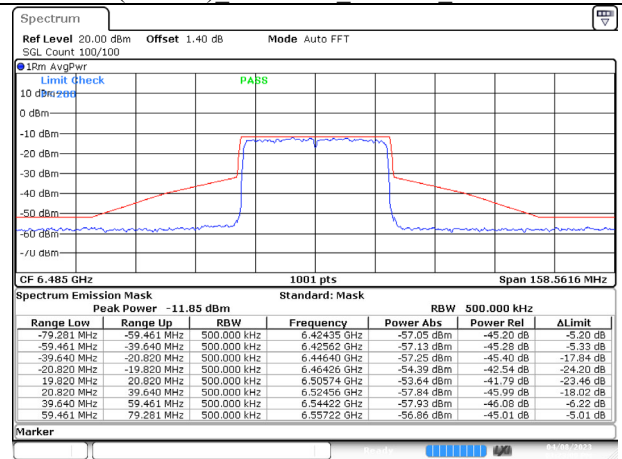
802.11ax (40MHz) 6485MHz Chain B NSS-1
