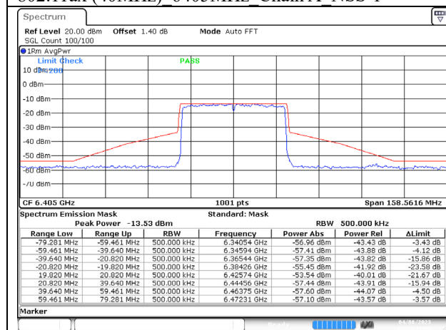
802.11ax (40MHz) 6405MHz Chain A NSS-1
