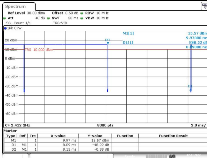
11B_Ant9_2412
