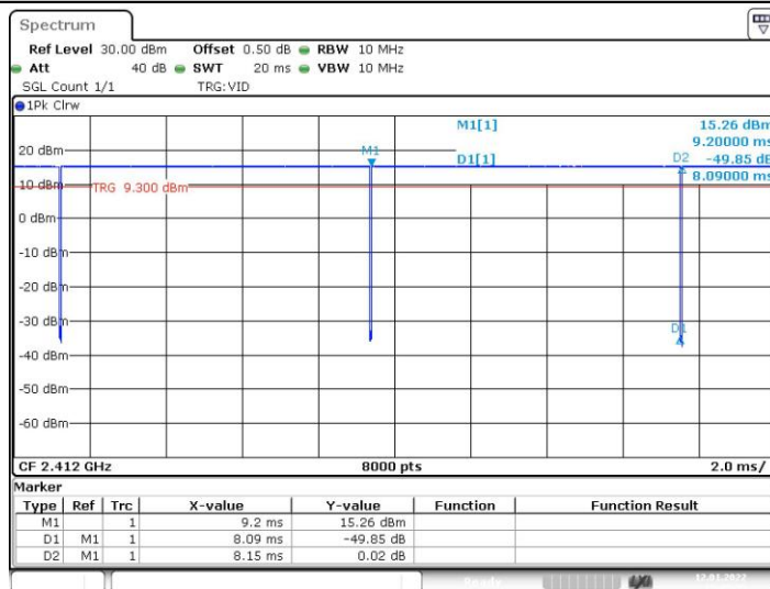
11B_Ant8_2412
