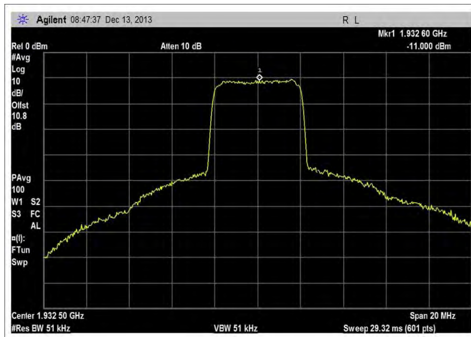
DL_1930-1995MHz_Output
