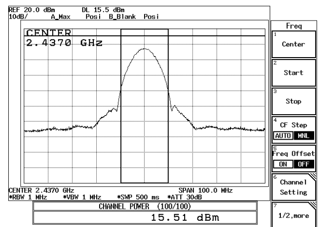
11Mbps-Ch06
