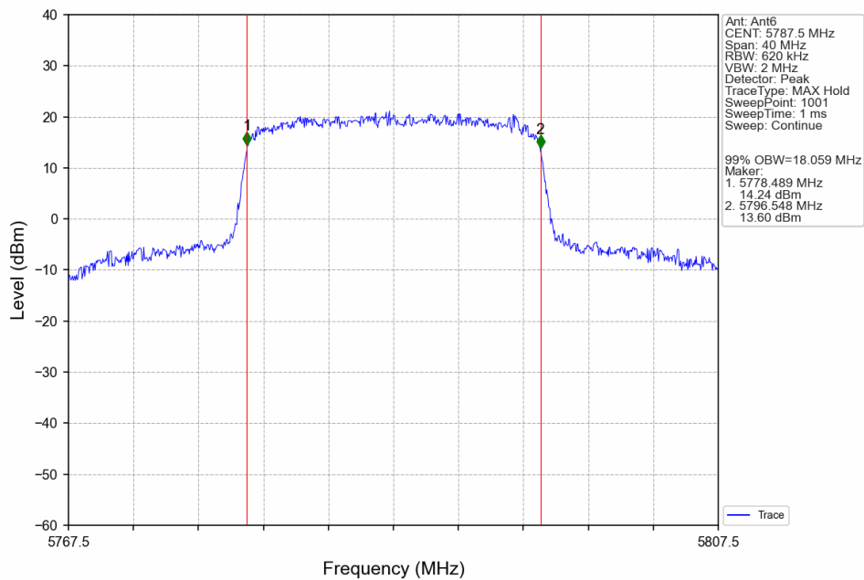
20M_MCH_5787.5MHz_Ant6_NTNV
