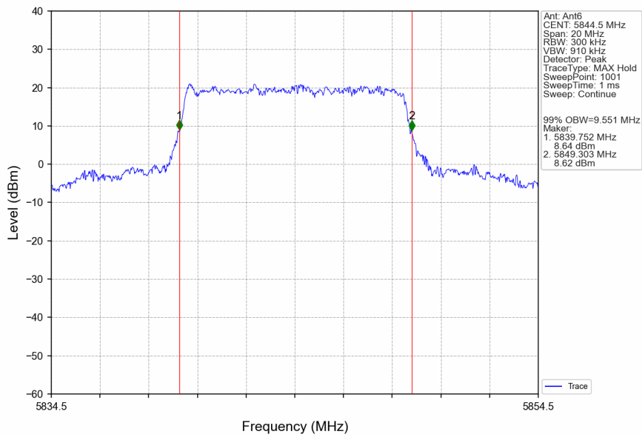
10M_HCH_5844.5MHz_Ant6_NTNV
