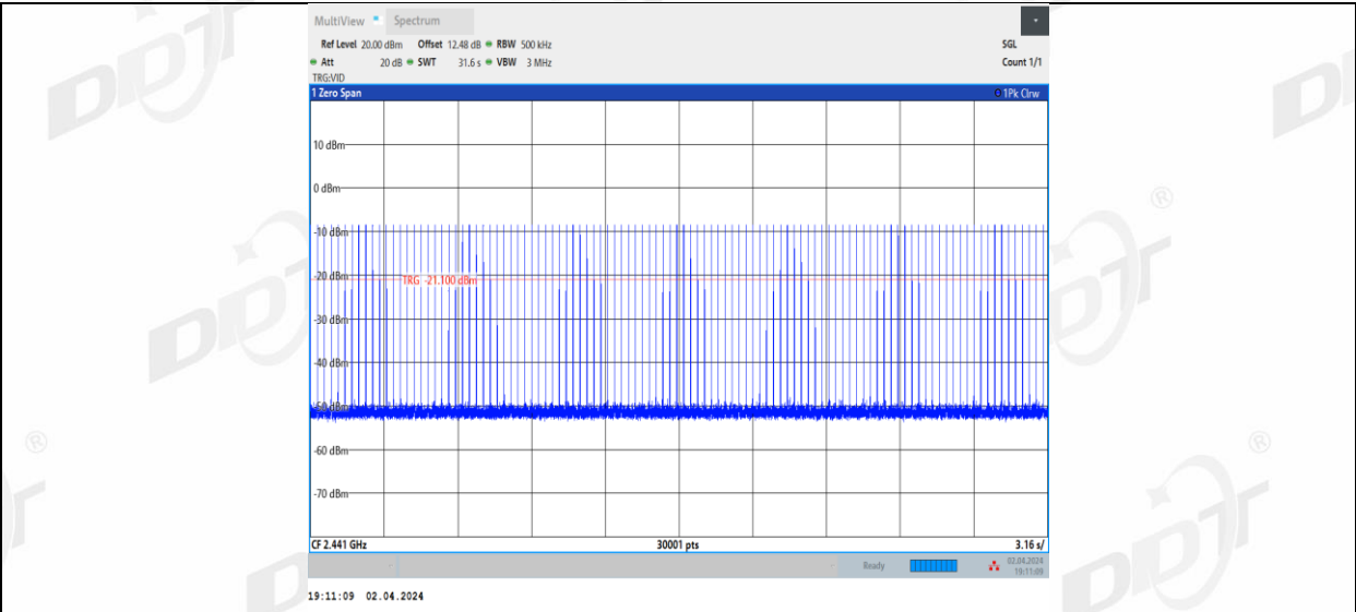
3DH5_Right side_Hop
