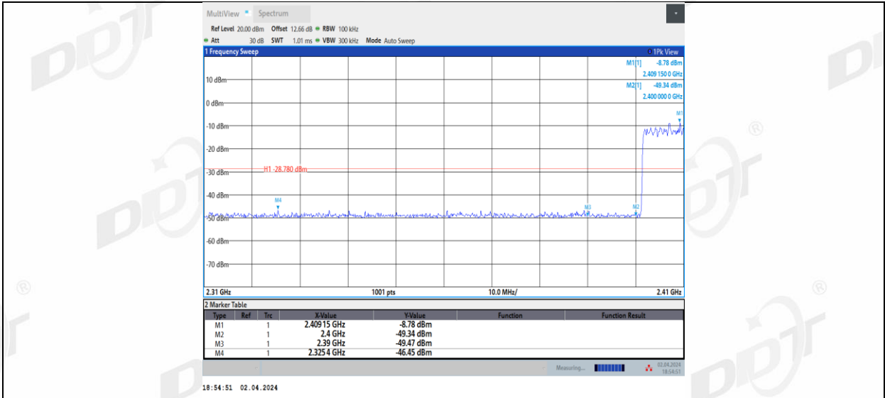
2DH5_Right side_Low_Hop_2402
