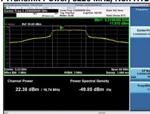
Antenna A
