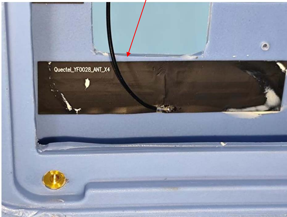
WWAN Antenna 2
