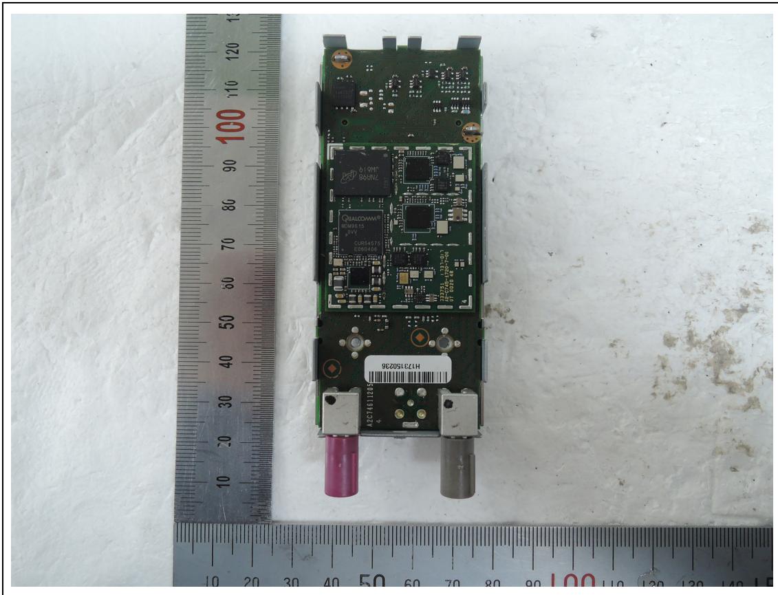
<LTE Module>
