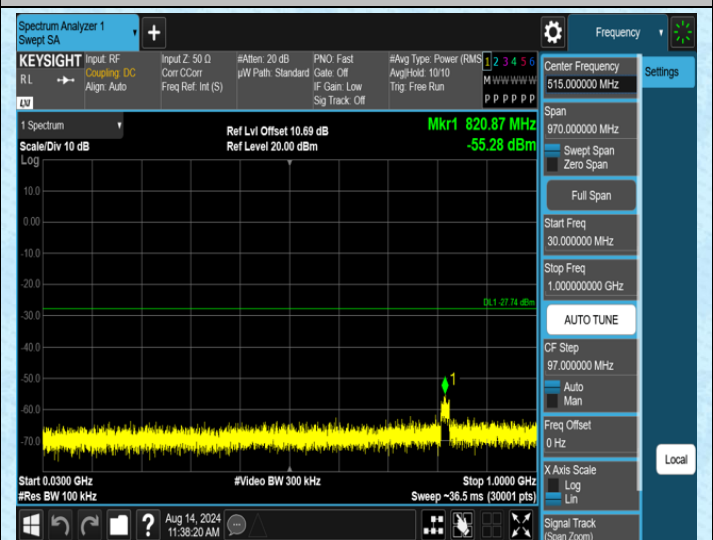
11G-Ant1-2462-30~1000
