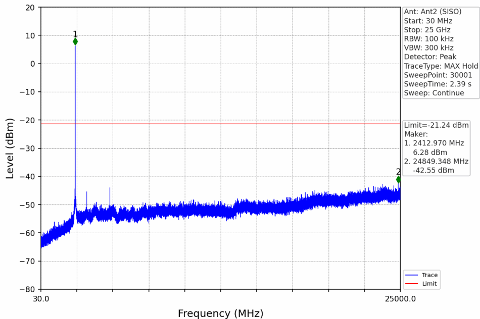
802.11b_LCH_2412MHz_Ant2 (SISO)_NTNV
