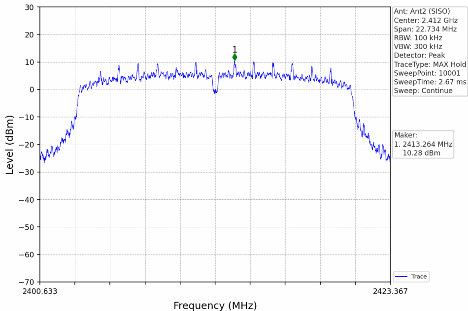
802.11n(HT20)_LCH_2412MHz_Ant2 (SISO)_NTNV
