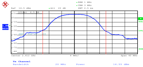
802.11b
