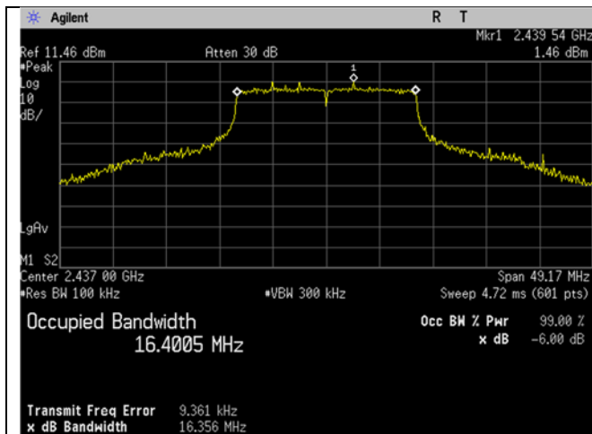
2437MHz_g-mode_-6dB
