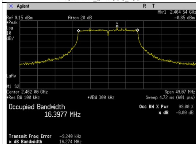
2462MHz_g-mode_-6dB
