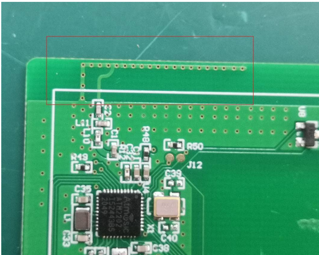
Antenna
