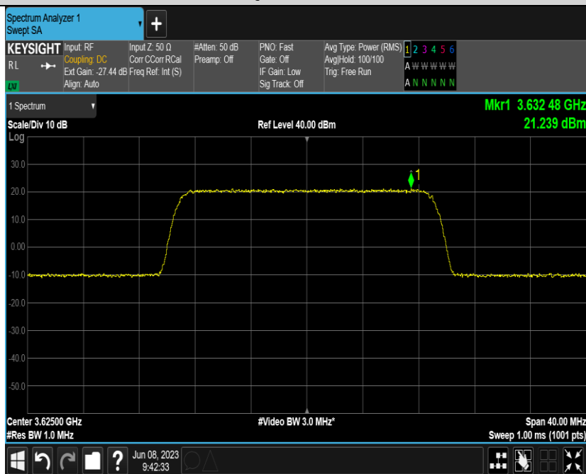
Band48-20MHz-QPSK-56640-E-TM1.1-1000
