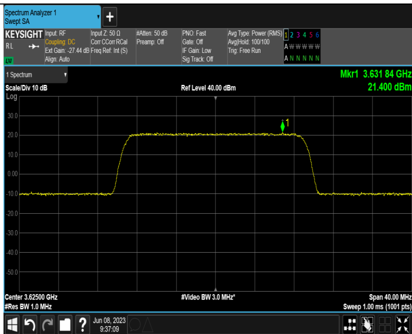
Band48-20MHz-QPSK-56640-E-TM1.1-1000
