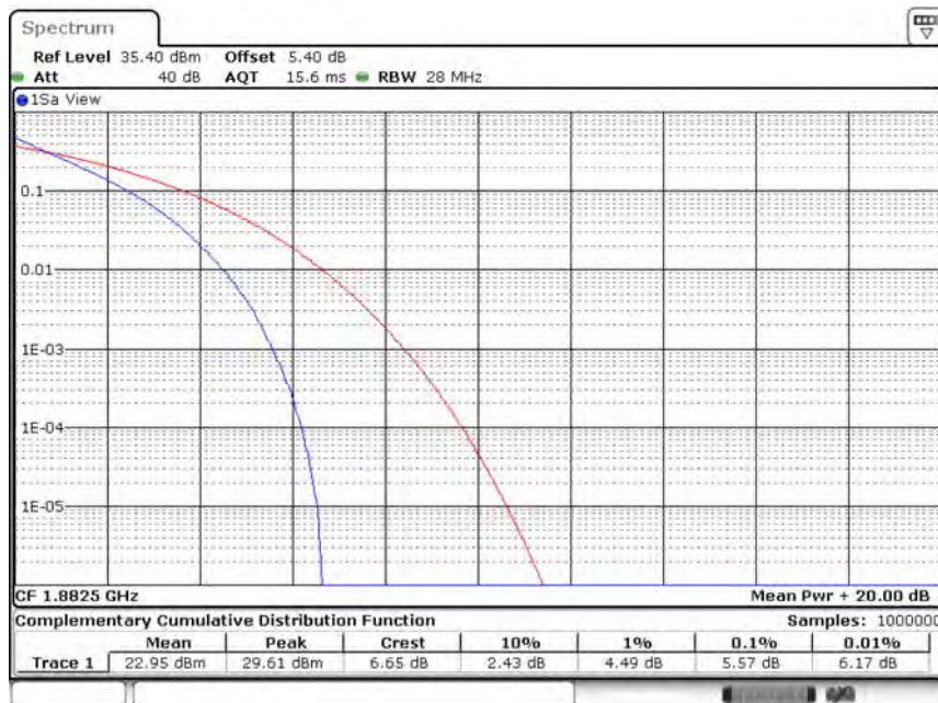
Band25-20MHz-QPSK-26365-100RB#0
