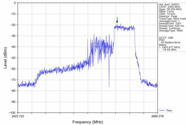
802.11ax(HEW40)_HCH_2452MHz_RU242_62_Ant1 (SISO)_NTNV
