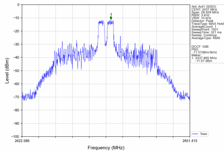
802.11ax(HEW20)_MCH_2437MHz_RU52_38_Ant1 (SISO)_NTNV
