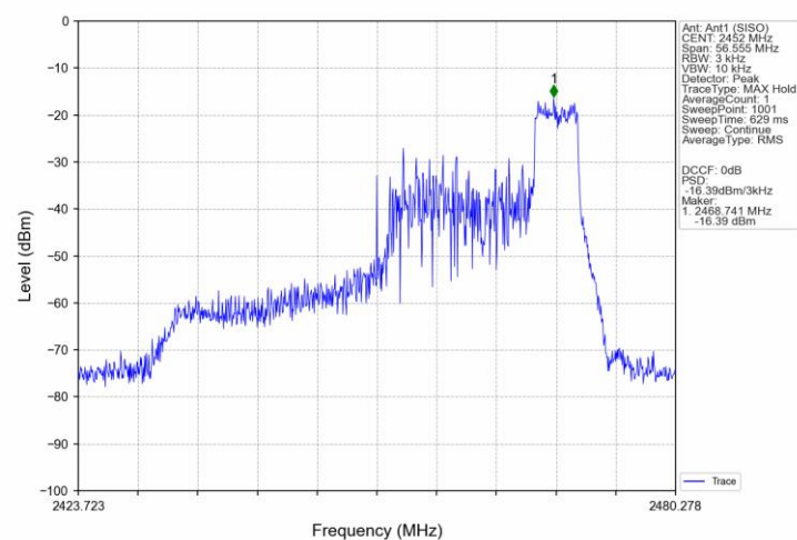
802.11ax(HEW40)_HCH_2452MHz_RU106_56_Ant1 (SISO)_NTNV
