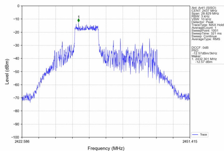
802.11ax(HEW20)_MCH_2437MHz_RU106_53_Ant1 (SISO)_NTNV
