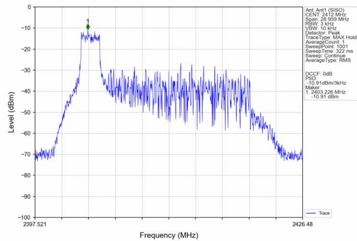
802.11ax(HEW20)_LCH_2412MHz_RU52_37_Ant1 (SISO)_NTNV
