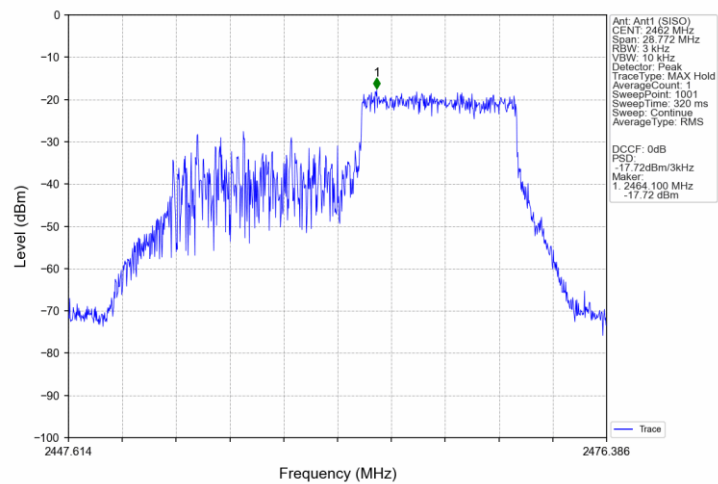
802.11ax(HEW20)_HCH_2462MHz_RU242_61_Ant1 (SISO)_NTNV
