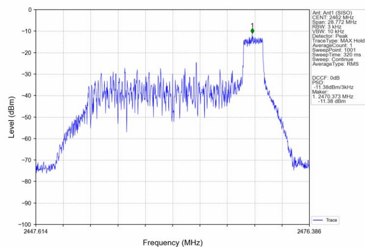
802.11ax(HEW20)_HCH_2462MHz_RU52_40_Ant1 (SISO)_NTNV
