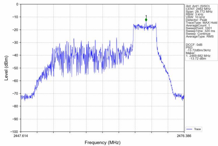
802.11ax(HEW20)_HCH_2462MHz_RU106_54_Ant1 (SISO)_NTNV
