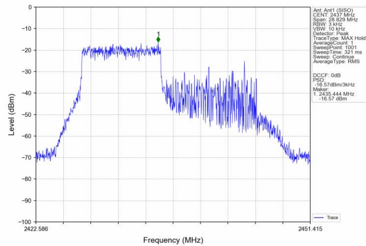
802.11ax(HEW20)_MCH_2437MHz_RU242_61_Ant1 (SISO)_NTNV
