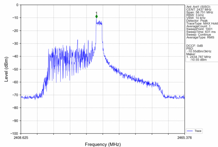
802.11ax(HEW40)_MCH_2437MHz_RU52_40_Ant1 (SISO)_NTNV
