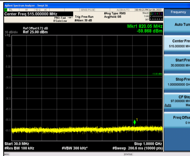
Band2-20MHz-QPSK-18900-1-0-Low-30-1000--59.87-PASS
