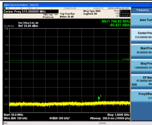
Band2-20MHz-QPSK-19100-1-0-Low-30-1000--60.42-PASS
