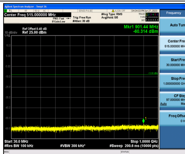
Band4-5MHz-QPSK-20375-1-0-Low-30-1000--60.31-PASS
