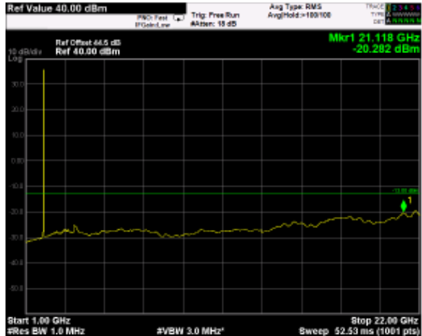
1GHz-22GHz
