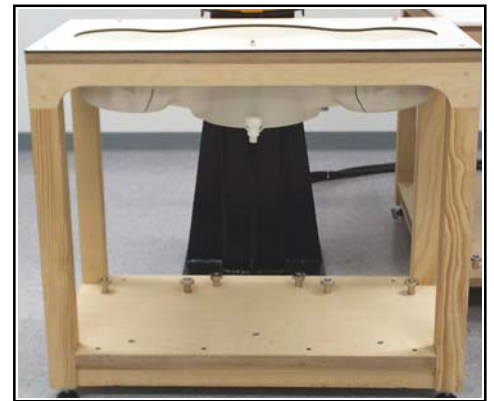
SAM Phantom
