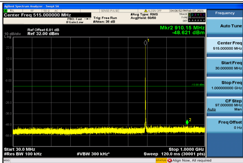
Band12-1.4MHz-QPSK-23017-1RB#0-30~1000MHz
