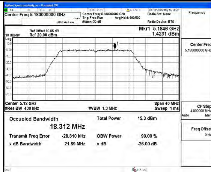
11AC20MIMO_Ant2_5180
