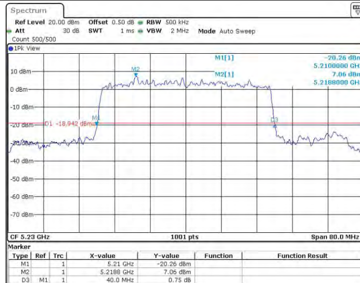
11AX40SISO_Ant0_5230
