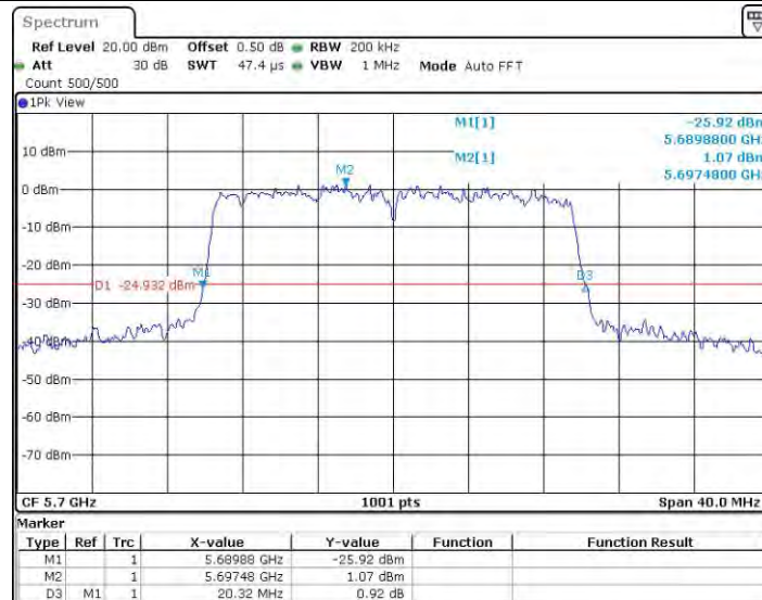
11AX20SISO_Ant1_5700
