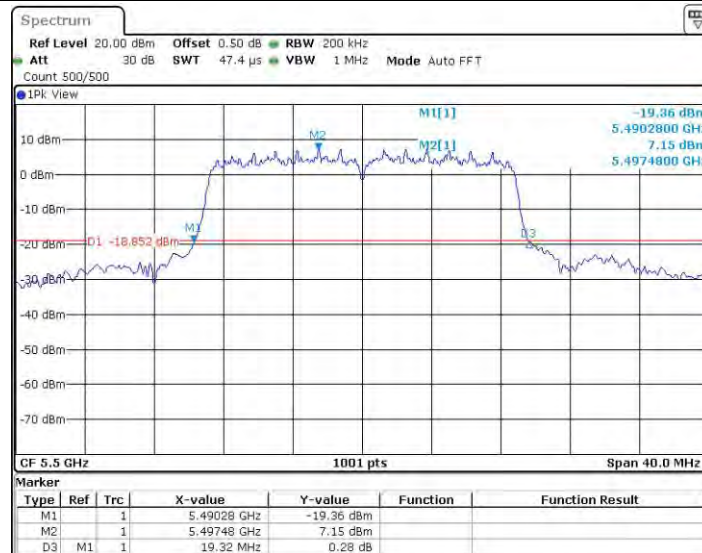
11N20SISO_Ant0_5500
