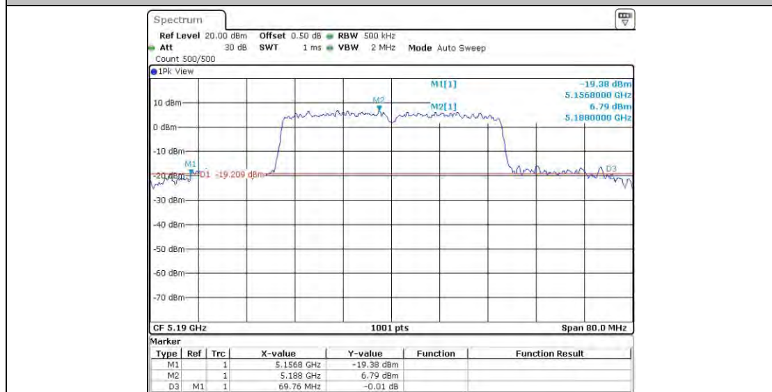
11N40SISO_Ant0_5190
