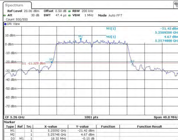
11A_Ant0_5260
