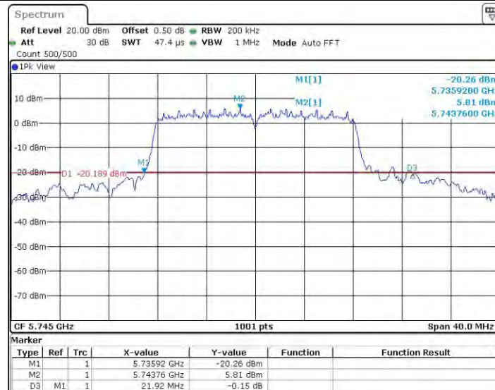
11A_Ant0_5745
