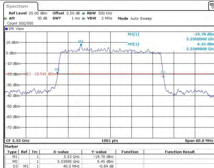
11AX40SISO_Ant1_5550
