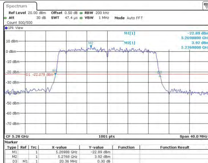
11AX20SISO_Ant0_5280
