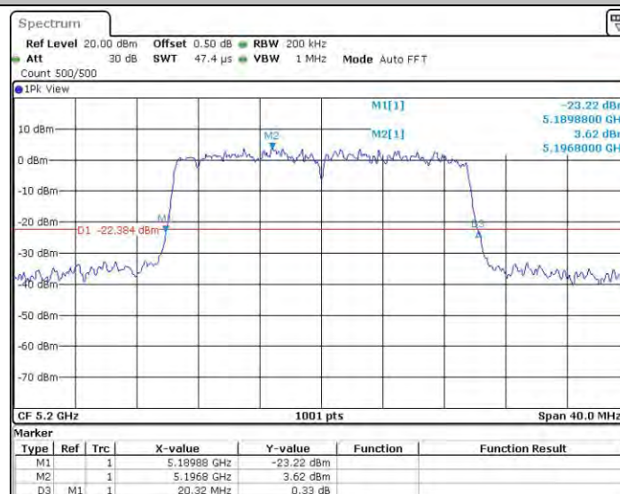
11AX20SISO_Ant0_5200
