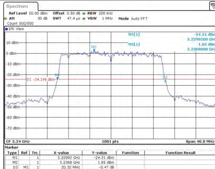
11N20MIMO_Ant0_5240
