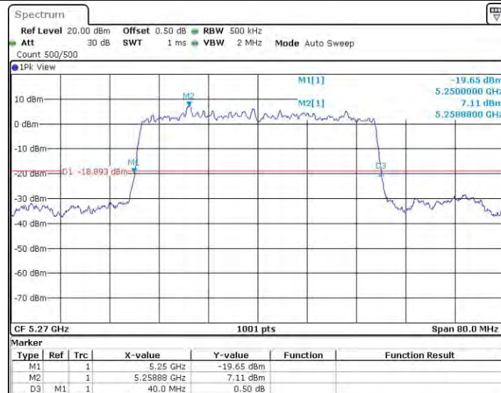
11AX40SISO_Ant1_5270
