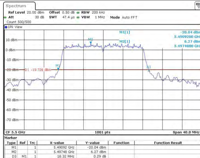
11A_Ant0_5500
