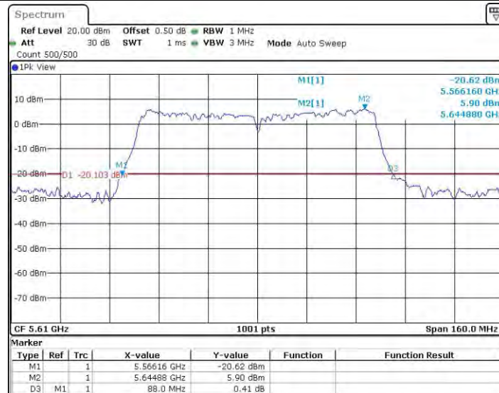
11AC80SISO_Ant0_5610
