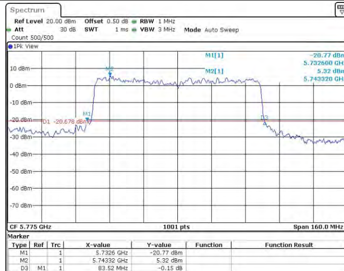
11AX80SISO_Ant0_5775
