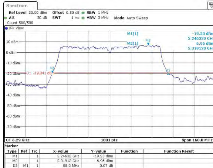
11AC80SISO_Ant0_5290
