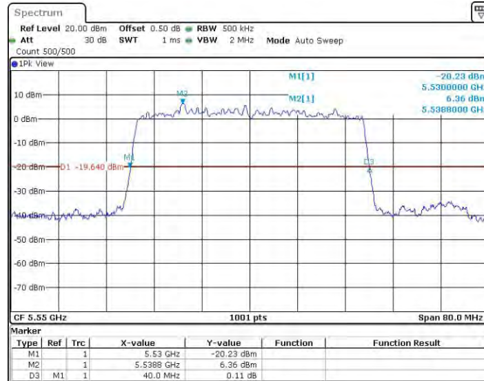
11AX40SISO_Ant0_5550
