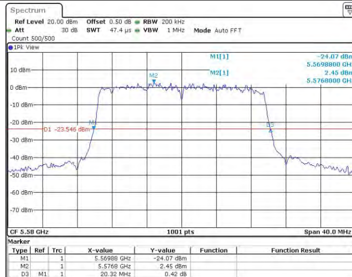
11AX20SISO_Ant0_5580
