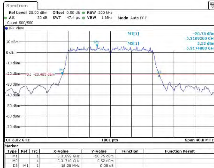
11A_Ant1_5320
