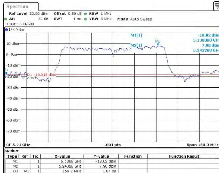
11AC80SISO_Ant0_5210
