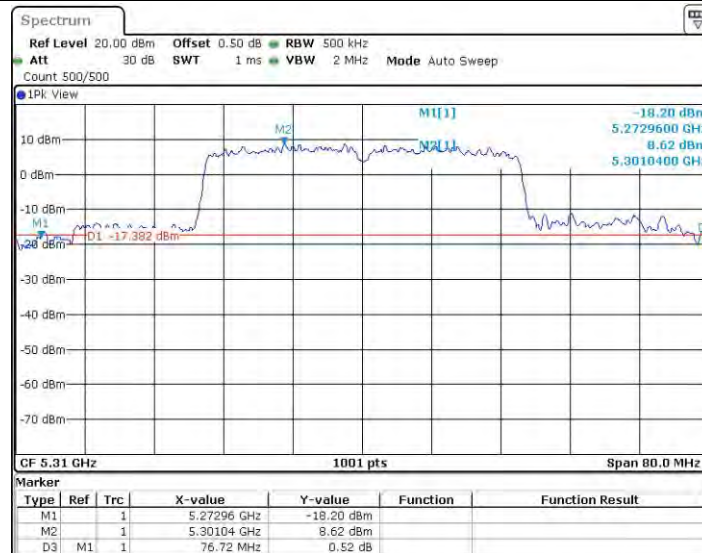
11N40SISO_Ant0_5310
