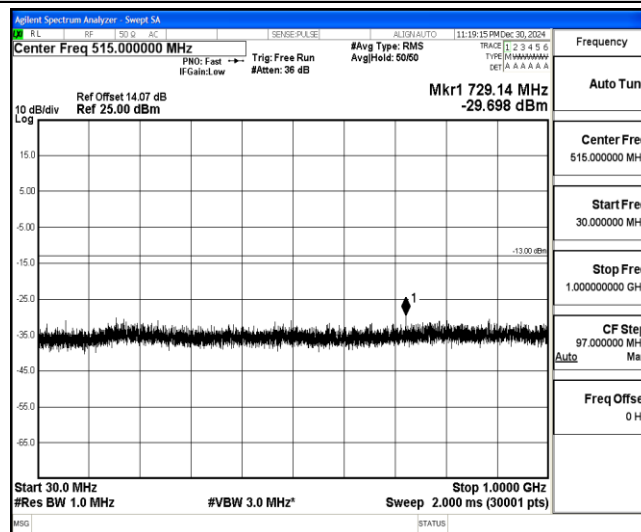
Band4-10MHz-QPSK-20000-1-0-Low-30-1000--29.7-PASS
