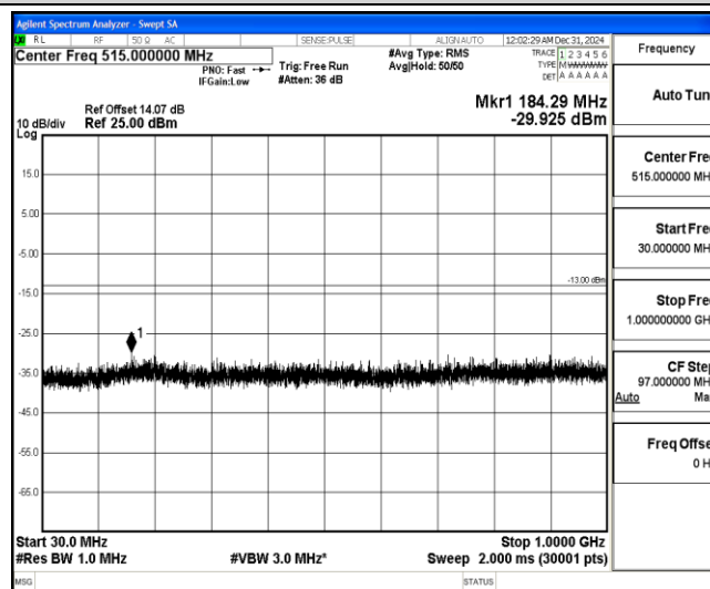
Band4-20MHz-QPSK-20050-1-0-Low-30-1000--29.93-PASS
