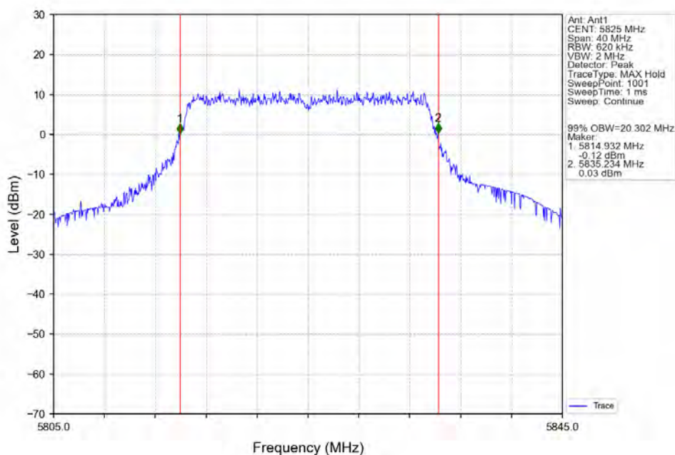
802.11ax(HE20)_HCH_5825MHz_RU242_Left_Ant1_NTNV
