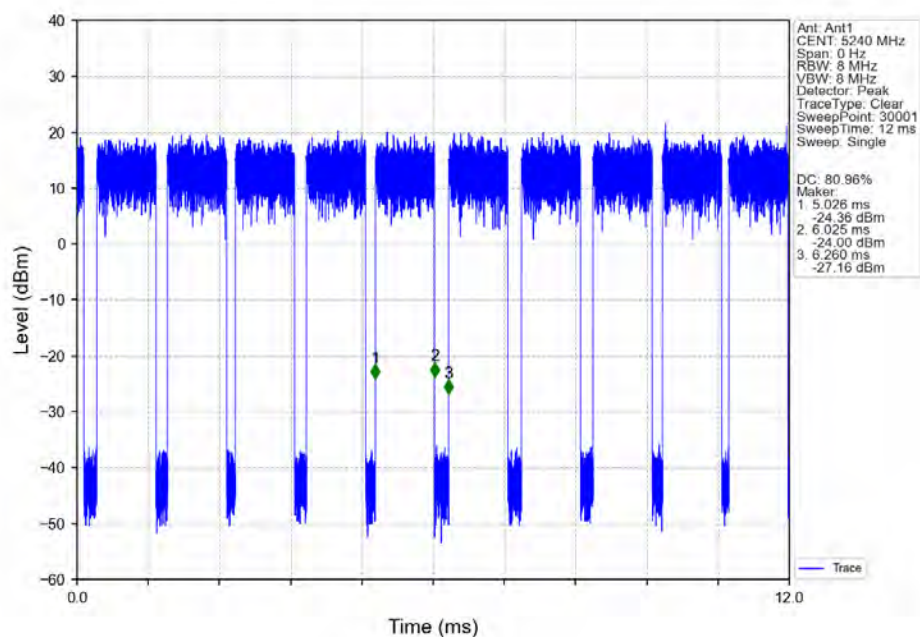
802.11ax(HE20)_HCH_5240MHz_RU242_Left_Ant1_NTNV
