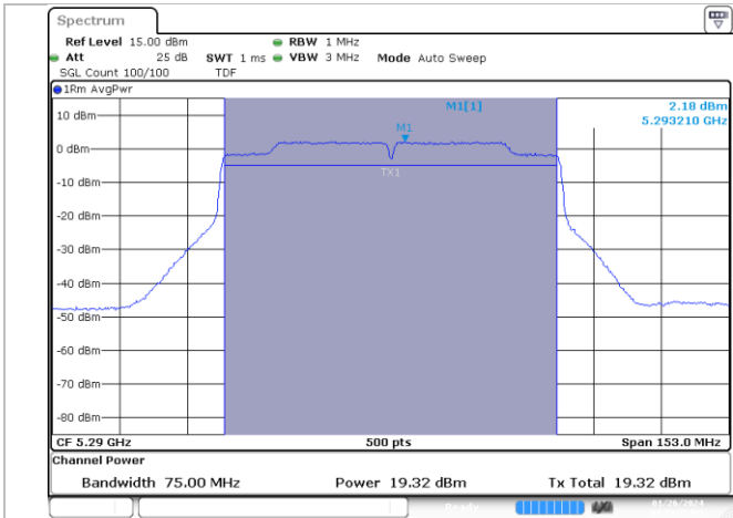
MIMO A-802.11ac-80MHz-Ch58-5290MHz-VHT0
