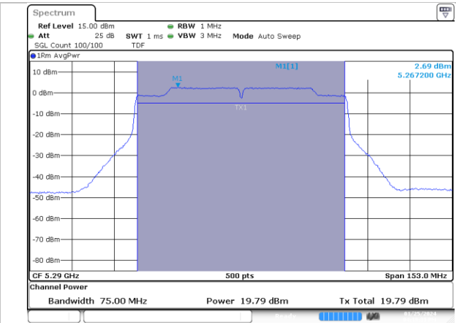
MIMO B-802.11ac-80MHz-Ch58-5290MHz-VHT0
