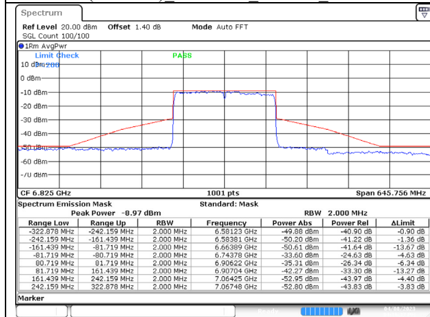
802.11ax (160MHz) 6825MHz Chain A NSS-1
