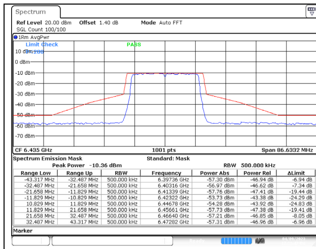
802.11ax (20MHz) 6435MHz Chain A NSS-4
