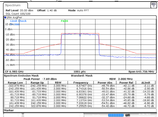
802.11ax (160MHz) 6985MHz Chain B NSS-1
