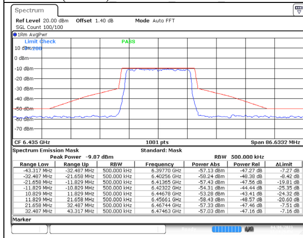
802.11ax (20MHz) 6435MHz Chain C NSS-4
