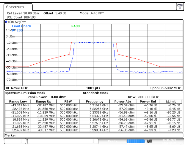
802.11ax (20MHz) 6255MHz Chain D NSS-4
