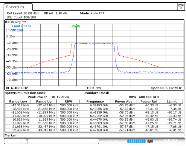
802.11ax (20MHz) 6435MHz Chain B NSS-4
