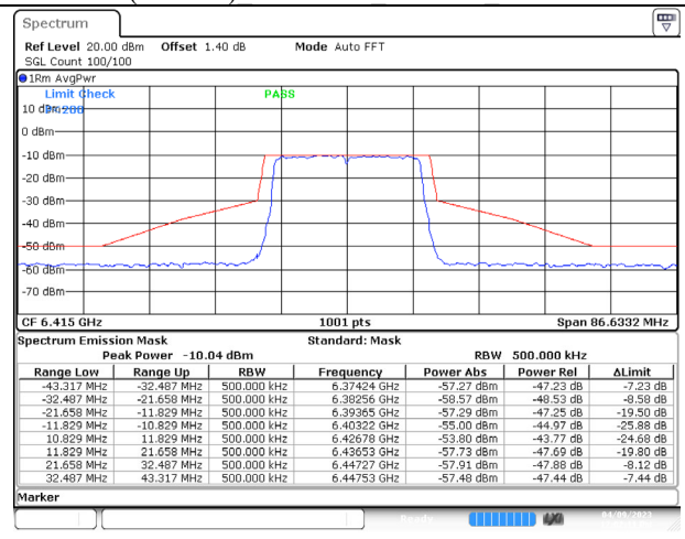
802.11ax (20MHz) 6415MHz Chain B NSS-4
