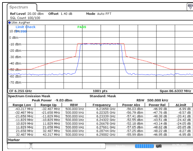
802.11ax (20MHz) 6255MHz Chain C NSS-4
