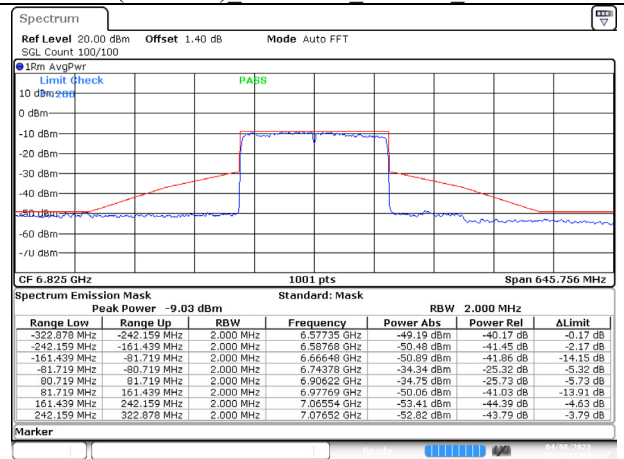
802.11ax (160MHz) 6825MHz Chain B NSS-1
