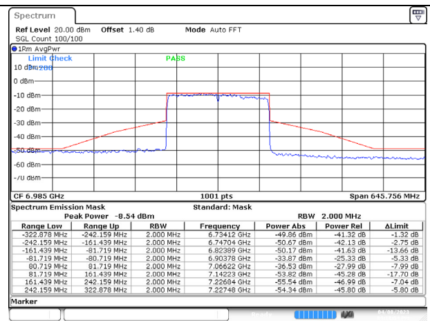
802.11ax (160MHz) 6985MHz Chain B NSS-1
