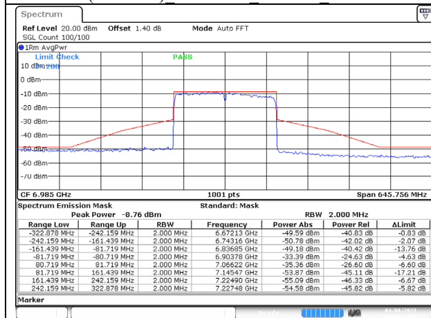
802.11ax (160MHz) 6985MHz Chain A NSS-1
