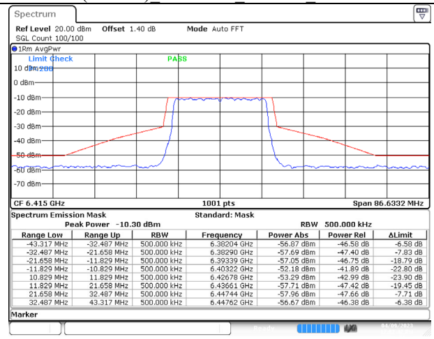
802.11ax (20MHz) 6415MHz Chain D NSS-4
