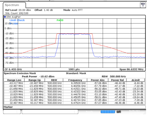
802.11ax (20MHz) 6435MHz Chain D NSS-4
