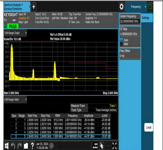
Band38_20MHz_QPSK_38150_1RB#0
