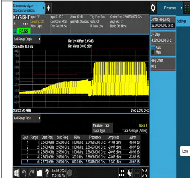
Band38_20MHz_QPSK_37850_100RB#0
