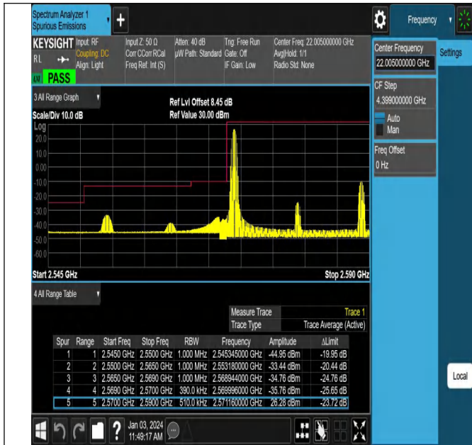
Band38_20MHz_QPSK_37850_1RB#0
