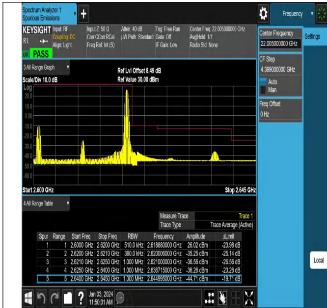
Band38_20MHz_QPSK_38150_1RB#99
