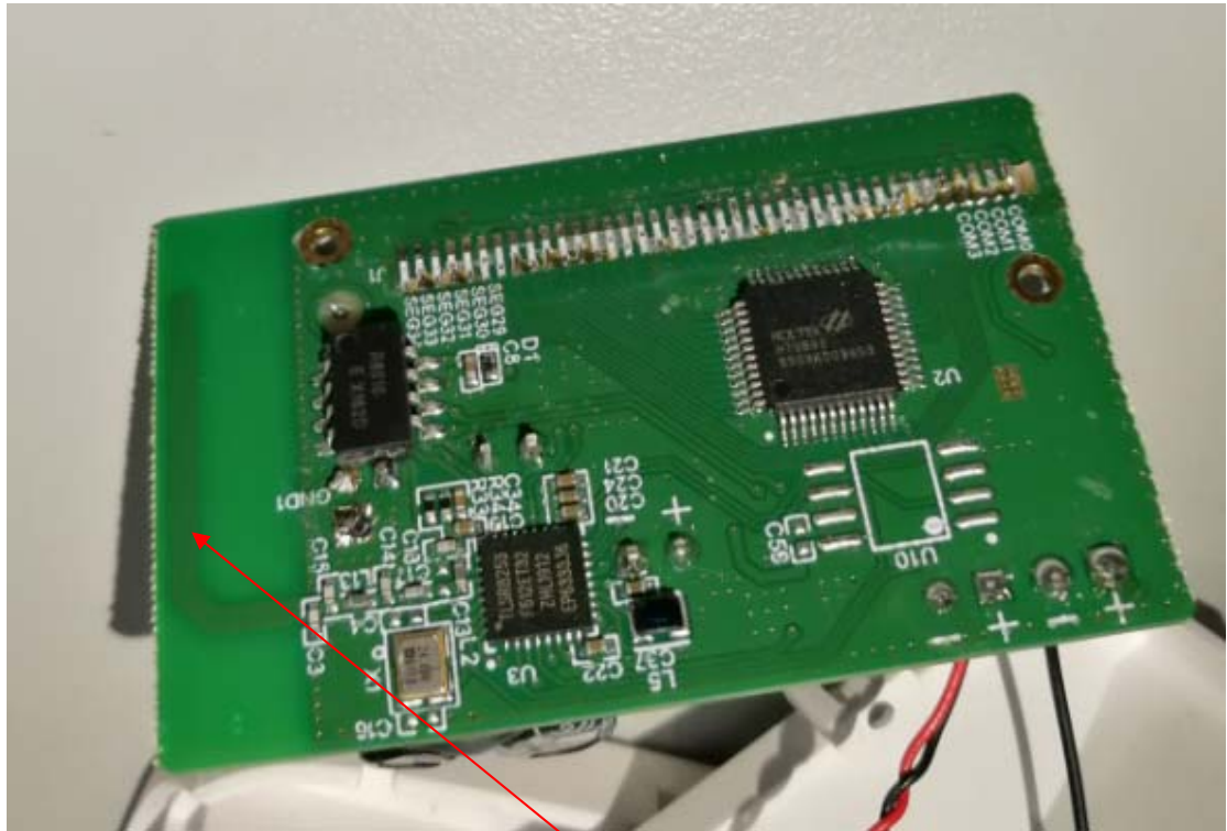
Antenna
