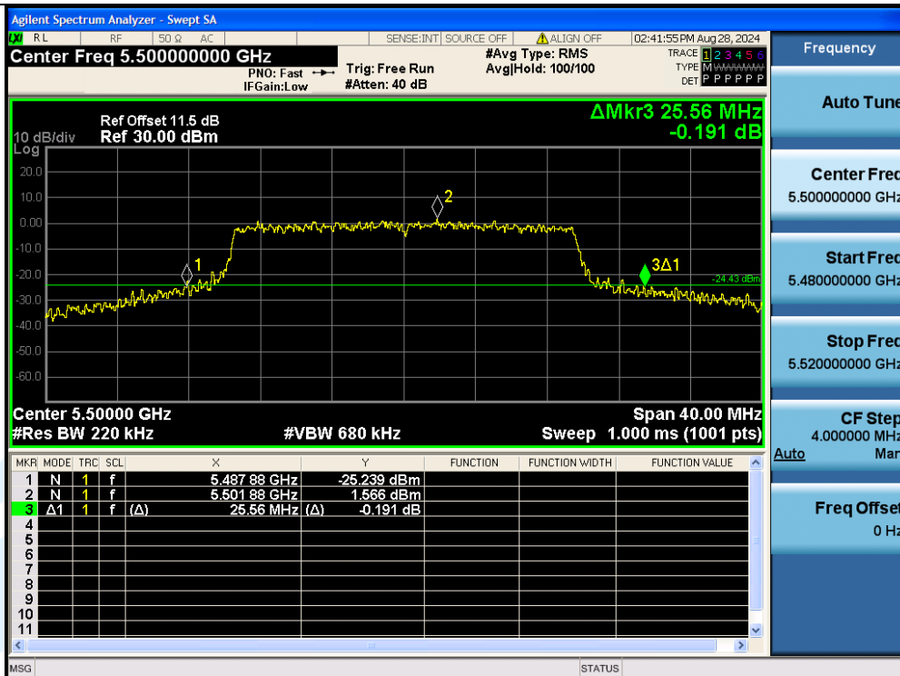
11AX20MIMO-Ant3-5500
