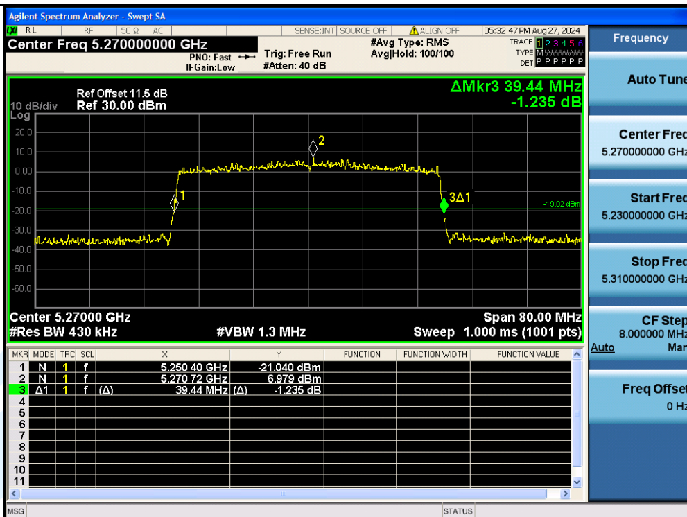
11AX40MIMO-Ant3-5270
