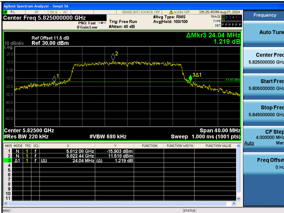
11AX20MIMO-Ant3-5825
