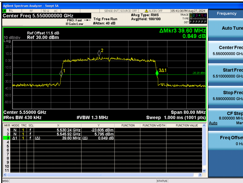
11AX40MIMO-Ant3-5550
