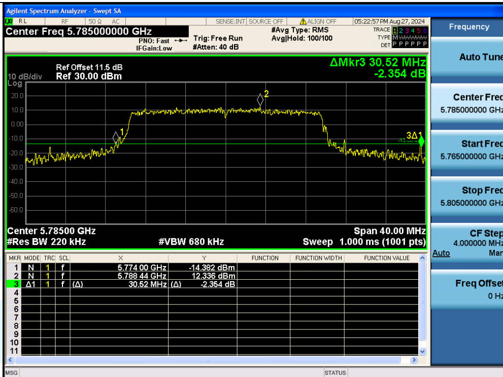
11AX20MIMO-Ant3-5785
