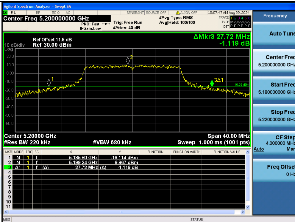
11A-Ant3-5200
