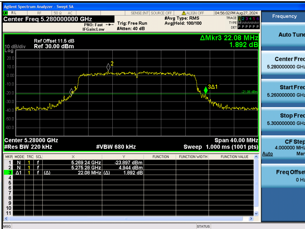
11AX20MIMO-Ant3-5280
