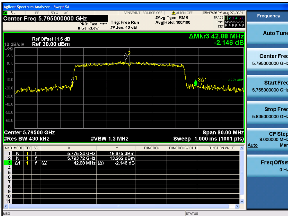
11AX40MIMO-Ant3-5795
