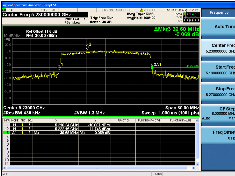
11AX40MIMO-Ant3-5230
