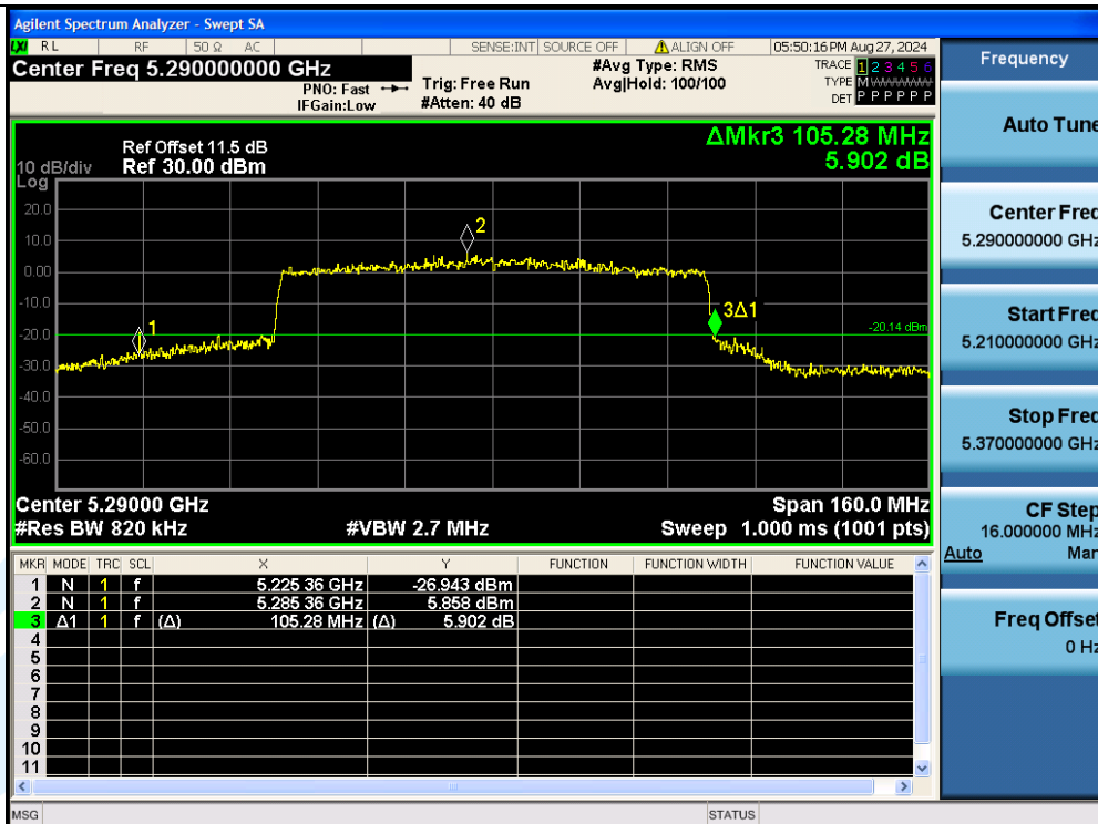
11AX80MIMO-Ant3-5290
