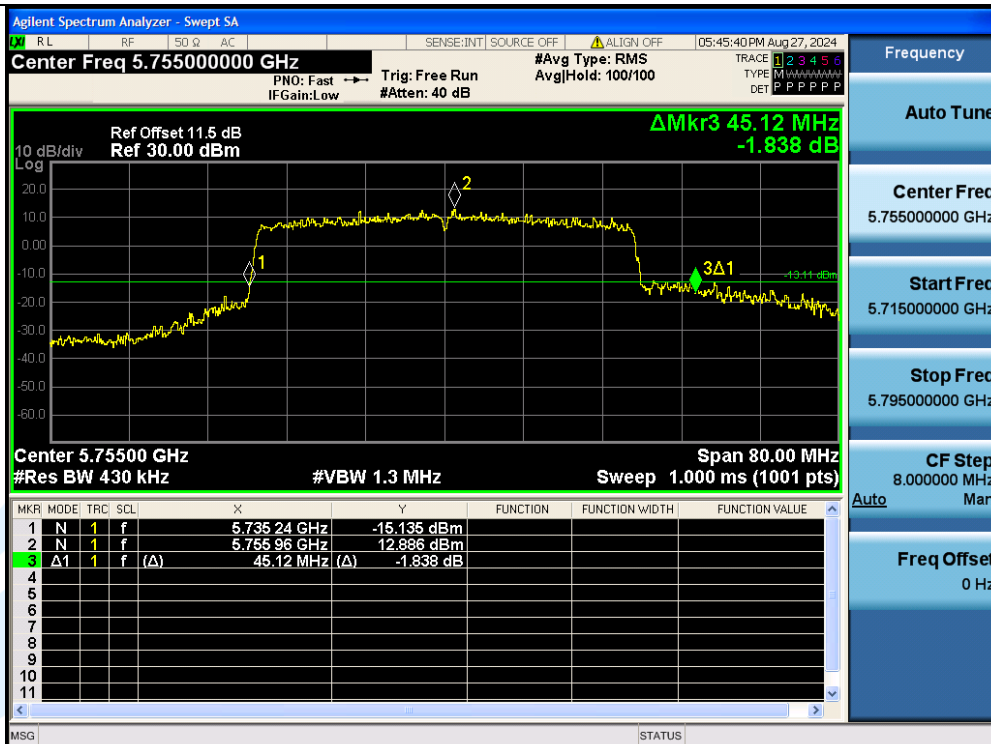
11AX40MIMO-Ant3-5755
