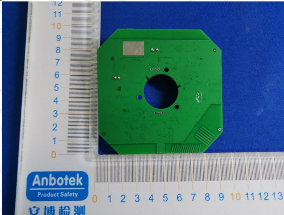
BT ANT
