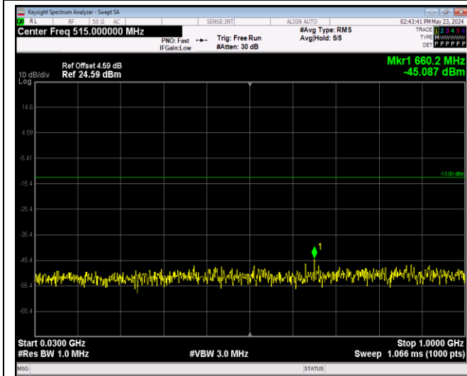
Band2-20MHz-QPSK-18700-1RB#0-Range1:30~1000MHz
