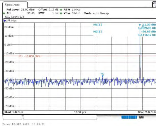
Band25-1.4MHz-QPSK-26365-1RB#0-Range2:1000~2000MHz
