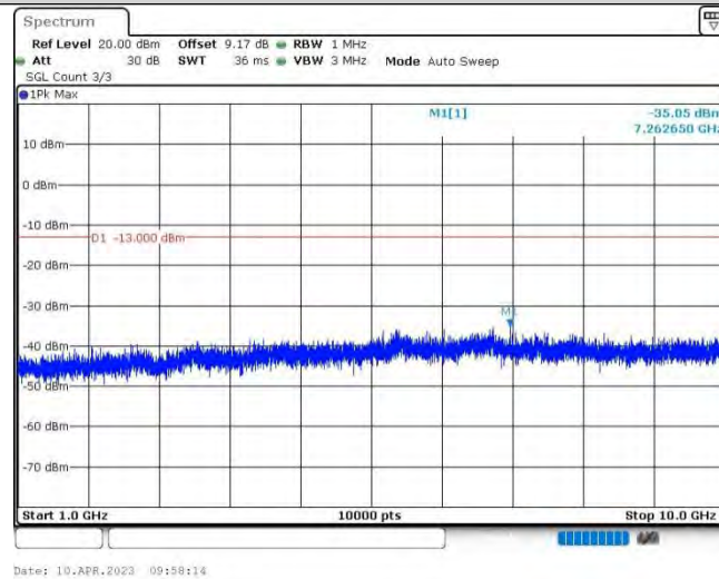
Band13-5MHz-QPSK-23255-1RB#0-Range2:1000~10000MHz
