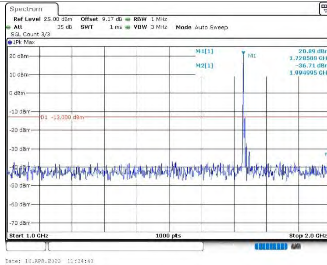
Band4-10MHz-QPSK-20175-1RB#0-Range2:1000~2000MHz
