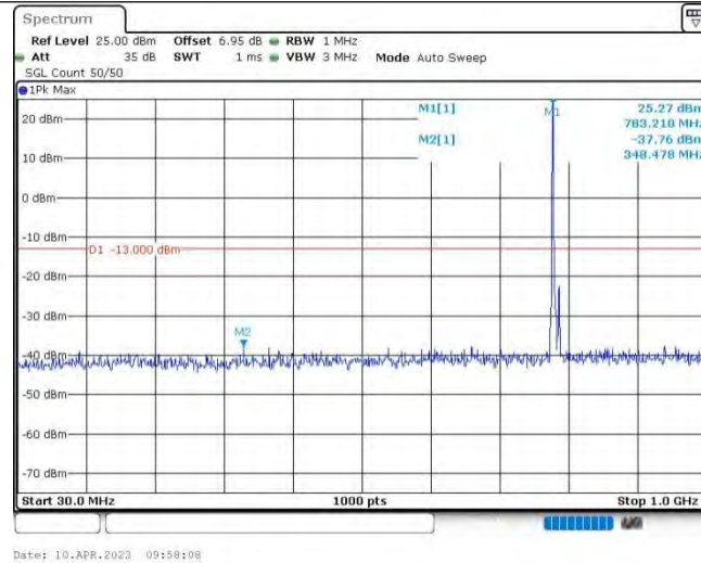
Band13-5MHz-QPSK-23255-1RB#0-Range1:30~1000MHz
