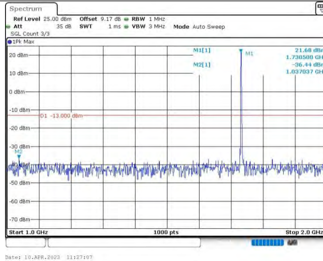
Band4-5MHz-QPSK-20175-1RB#0-Range2:1000~2000MHz
