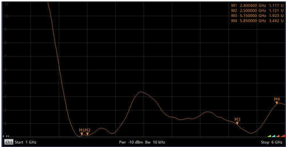
BT/WiFi Antenna
