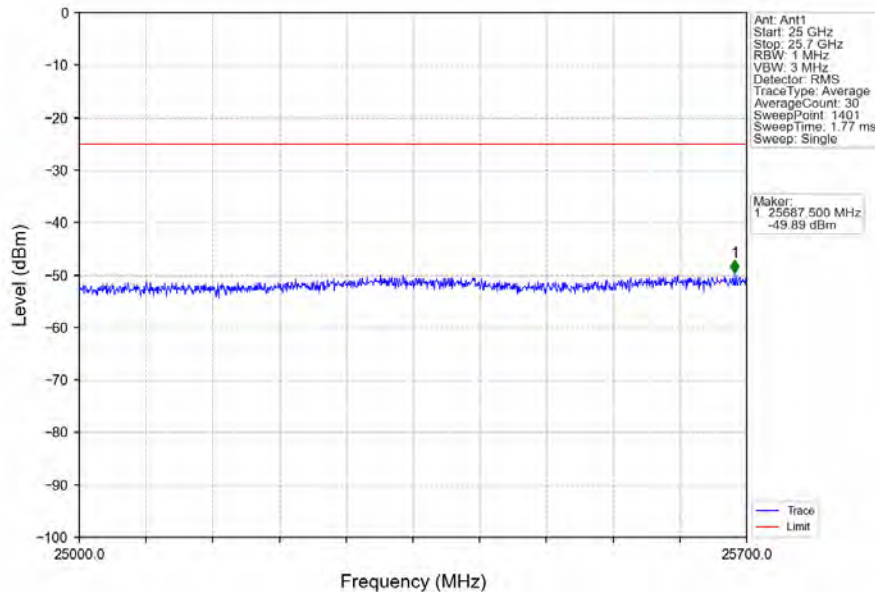
Band7_5MHz_QPSK_HCH_2567.5MHz_RB_1_24_NTNV
