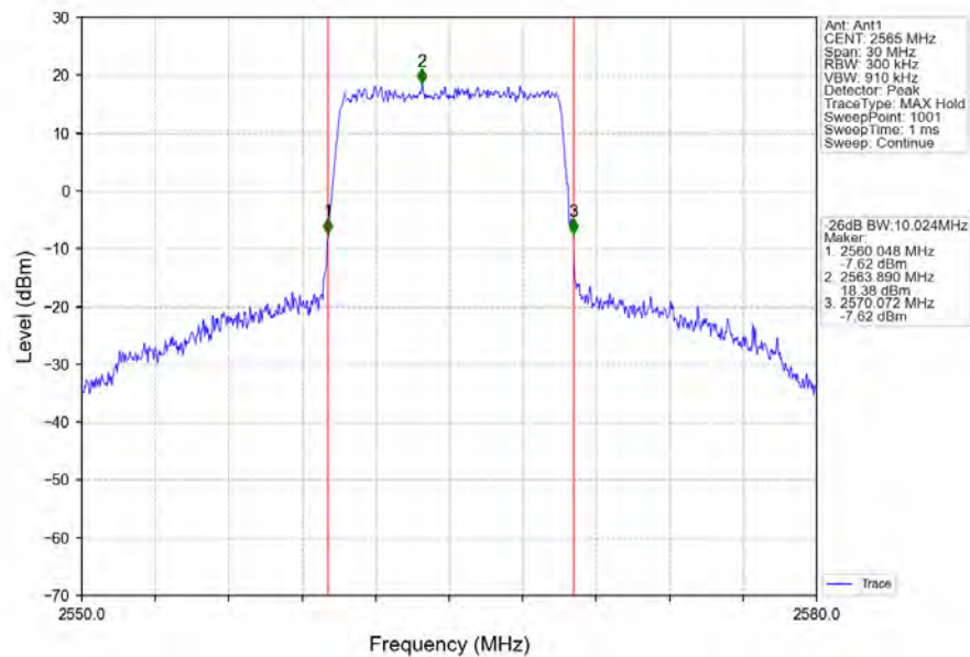
Band7_10MHz_QPSK_HCH_2565MHz_RB_50_0_NTNV
