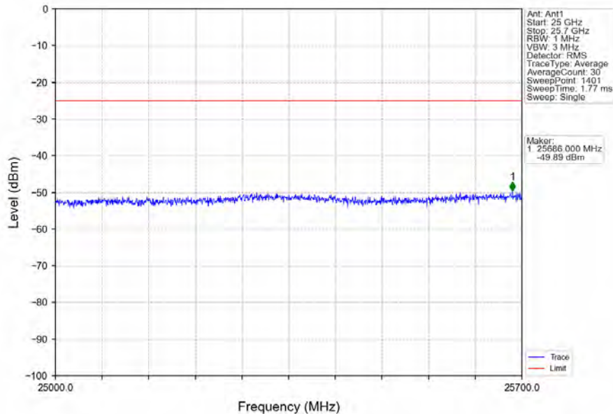
Band7_20MHz_16QAM_HCH_2560MHz_RB_1_0_NTNV
