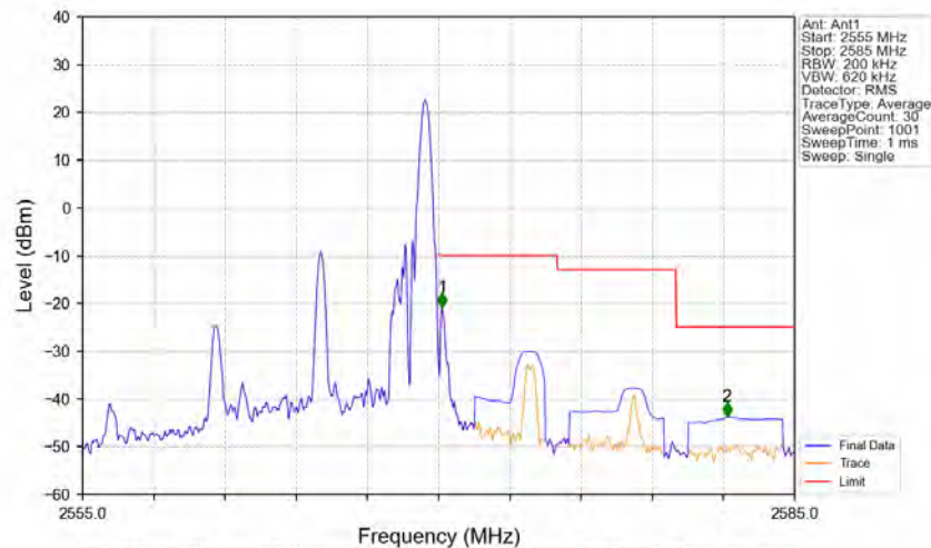
Band7_10MHz_QPSK_HCH_2565MHz_RB_1_49_NTNV
