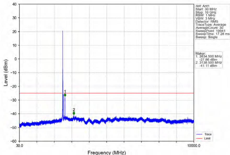
Band7_20MHz_64QAM_LCH_2510MHz_RB_1_0_NTNV
