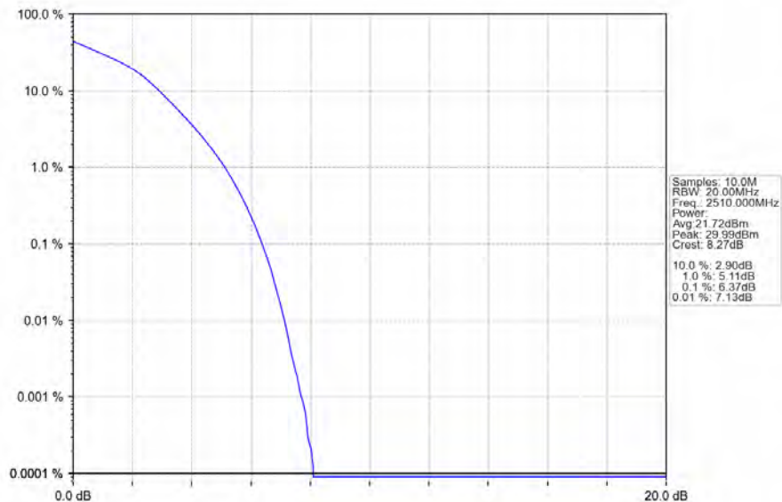
Band7_20MHz_16QAM_LCH_2510MHz_RB_100_0_NTNV
