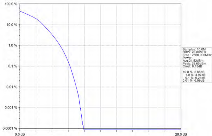
Band7_20MHz_16QAM_HCH_2560MHz_RB_100_0_NTNV
