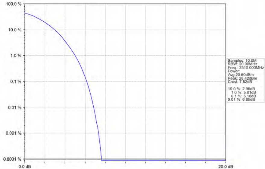
Band7_20MHz_64QAM_LCH_2510MHz_RB_100_0_NTNV
