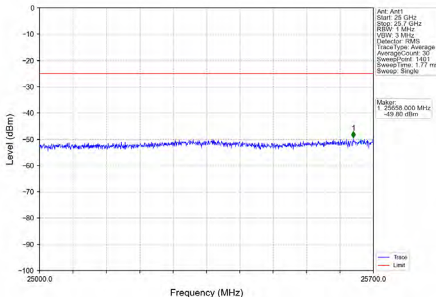
Band7_20MHz_64QAM_MCH_2535MHz_RB_1_0_NTNV
