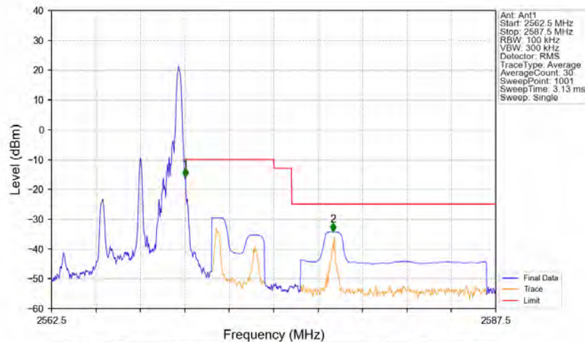
Band7_5MHz_QPSK_HCH_2567.5MHz_RB_1_24_NTNV
