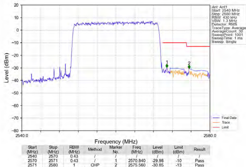
Band7_20MHz_16QAM_HCH_2560MHz_RB_100_0_NTNV
