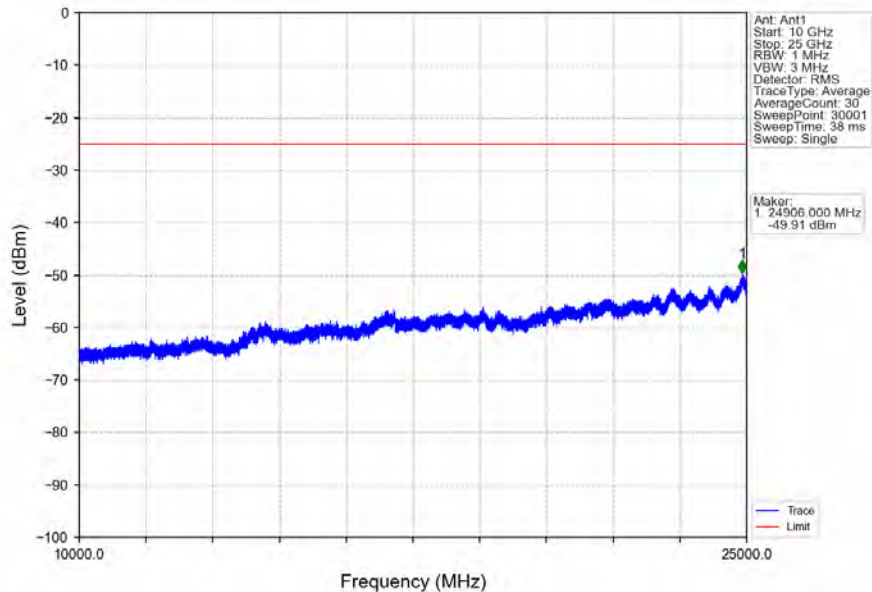
Band7_20MHz_64QAM_LCH_2510MHz_RB_1_0_NTNV
