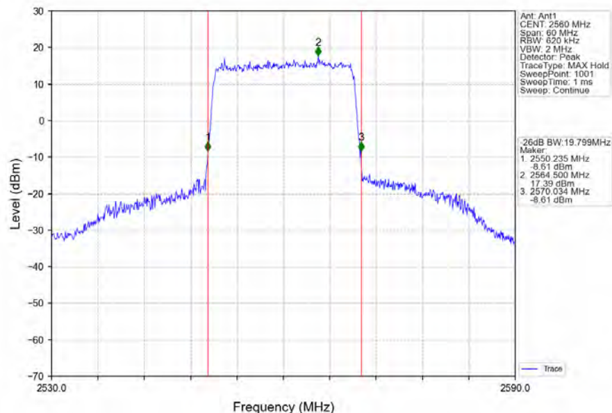
Band7_20MHz_64QAM_HCH_2560MHz_RB_100_0_NTNV
