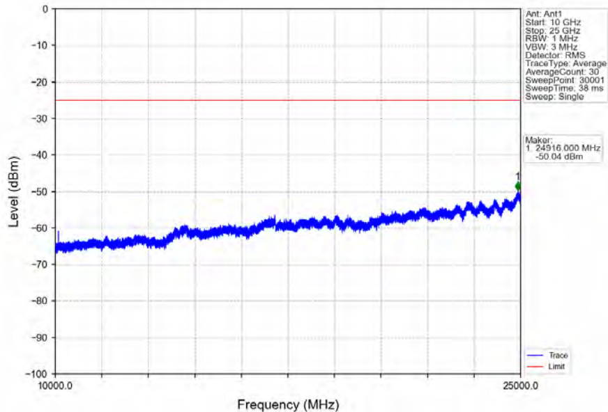
Band7_20MHz_QPSK_MCH_2535MHz_RB_1_0_NTNV
