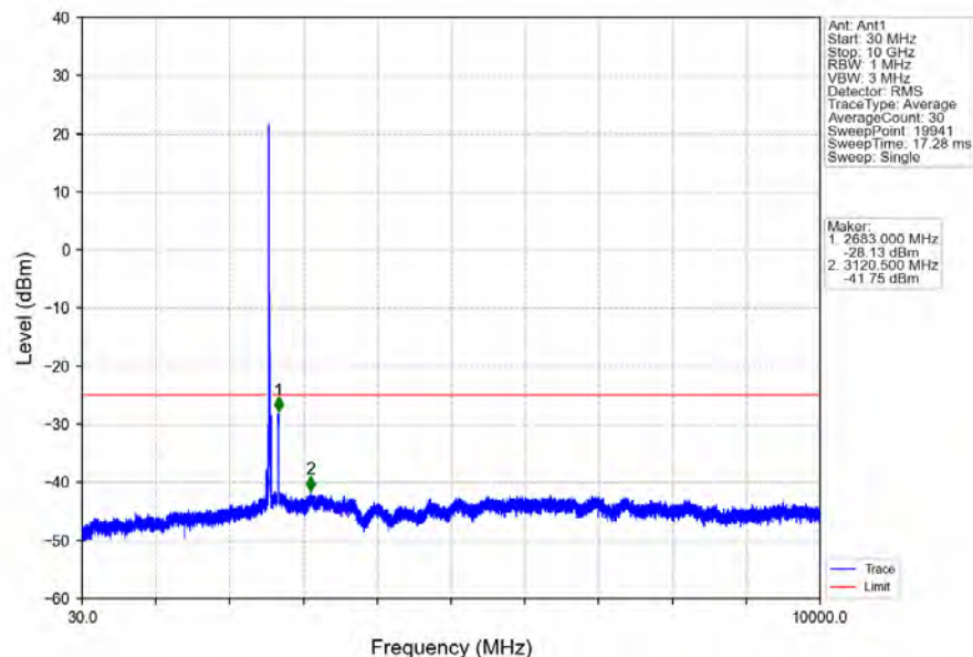
Band7_20MHz_16QAM_HCH_2560MHz_RB_1_0_NTNV
