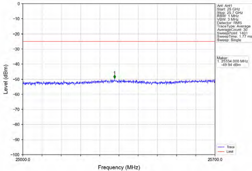
Band7_15MHz_QPSK_HCH_2562.5MHz_RB_1_74_NTNV
