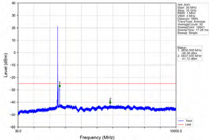
Band7_20MHz_16QAM_MCH_2535MHz_RB_1_0_NTNV
