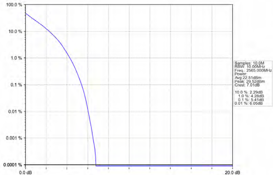
Band7_10MHz_QPSK_HCH_2565MHz_RB_50_0_NTNV
