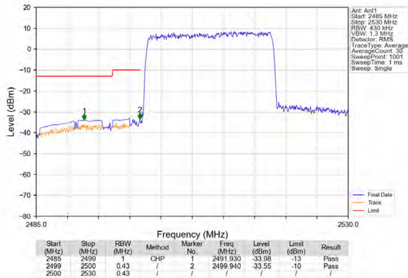
Band7_20MHz_QPSK_LCH_2510MHz_RB_100_0_NTNV
