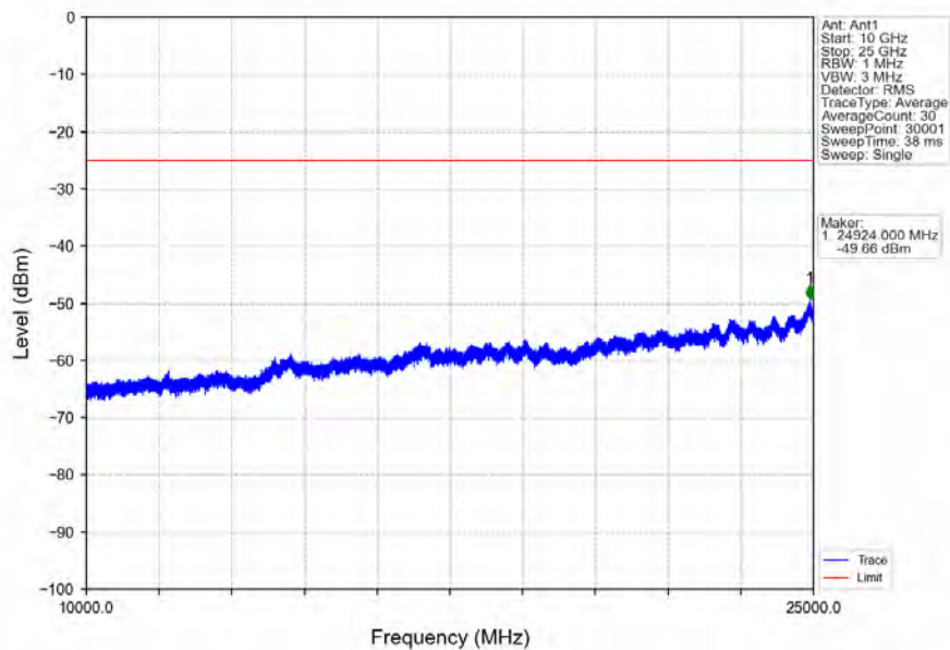
Band7_20MHz_16QAM_LCH_2510MHz_RB_1_0_NTNV
