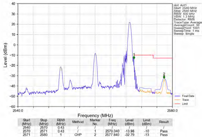
Band7_20MHz_16QAM_HCH_2560MHz_RB_1_99_NTNV
