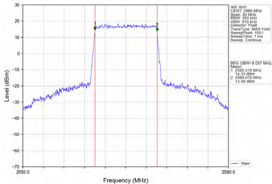
Band7_10MHz_QPSK_HCH_2565MHz_RB_50_0_NTNV
