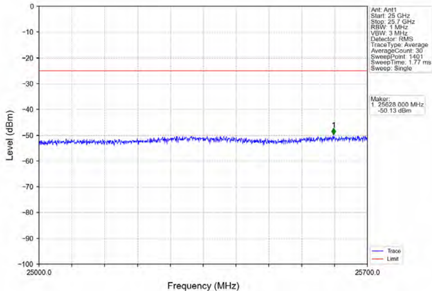
Band7_20MHz_64QAM_HCH_2560MHz_RB_1_99_NTNV
