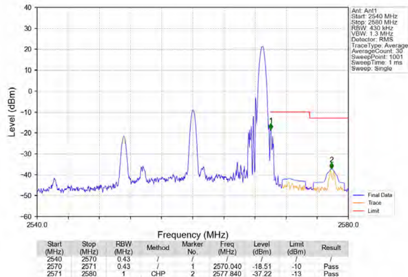
Band7_20MHz_64QAM_HCH_2560MHz_RB_1_99_NTNV
