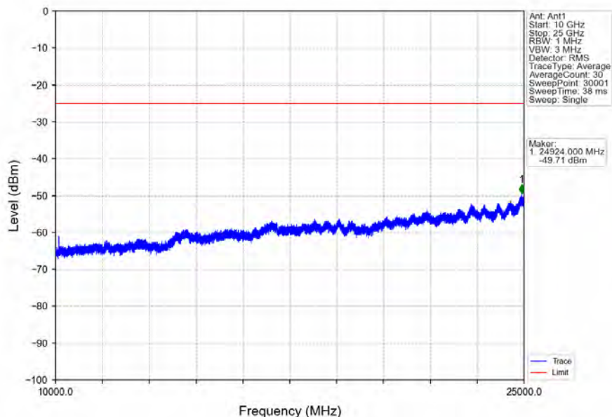
Band7_20MHz_16QAM_MCH_2535MHz_RB_1_0_NTNV
