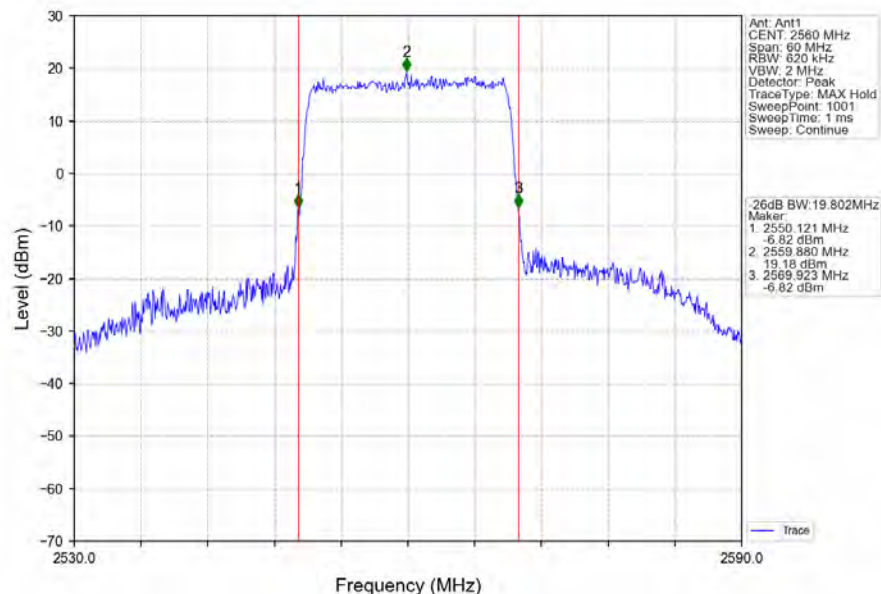
Band7_20MHz_QPSK_HCH_2560MHz_RB_100_0_NTNV
