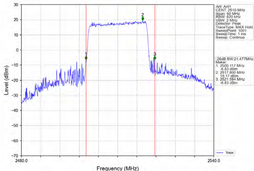
Band7_20MHz_QPSK_LCH_2510MHz_RB_100_0_NTNV
