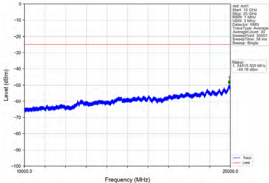
Band7_20MHz_QPSK_LCH_2510MHz_RB_1_0_NTNV
