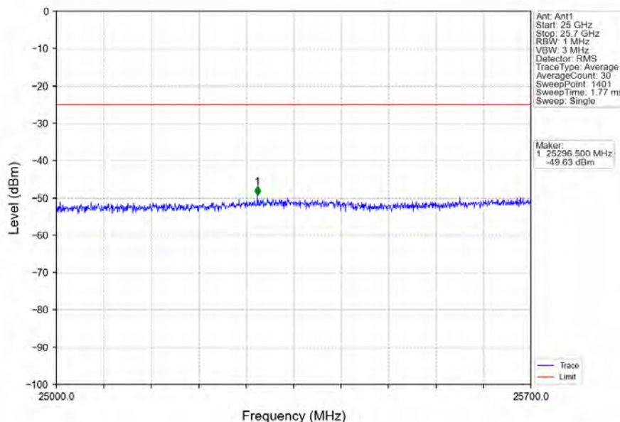
Band7_20MHz_16QAM_HCH_2560MHz_RB_1_0_NTNV
