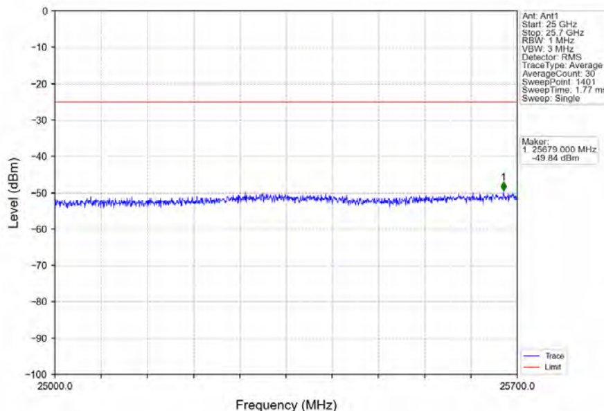
Band7_20MHz_64QAM_LCH_2510MHz_RB_1_0_NTNV
