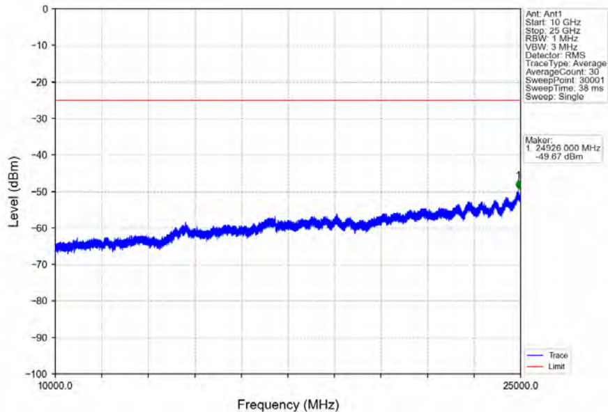
Band7_20MHz_16QAM_HCH_2560MHz_RB_1_0_NTNV
