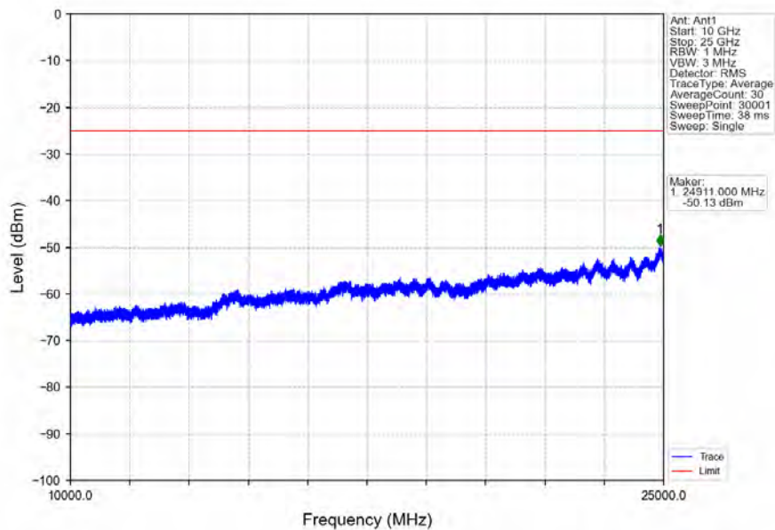
Band7_20MHz_64QAM_HCH_2560MHz_RB_1_0_NTNV
