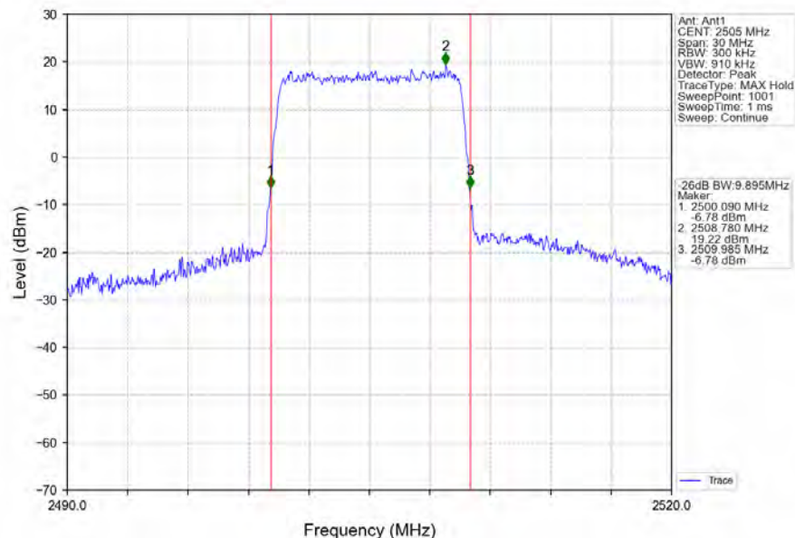
Band7_10MHz_QPSK_LCH_2505MHz_RB_50_0_NTNV
