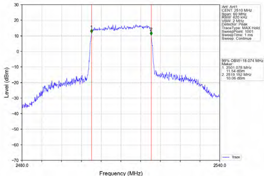
Band7_20MHz_64QAM_LCH_2510MHz_RB_100_0_NTNV
