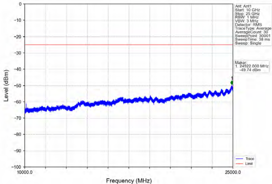
Band7_20MHz_64QAM_MCH_2535MHz_RB_1_0_NTNV
