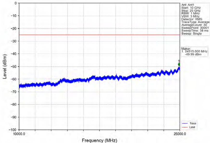
Band7_5MHz_QPSK_LCH_2502.5MHz_RB_1_0_NTNV
