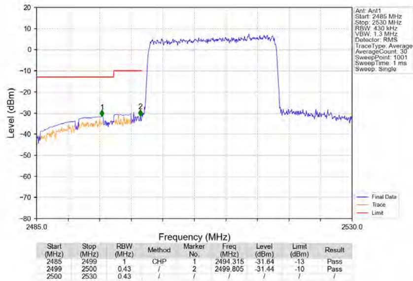
Band7_20MHz_64QAM_LCH_2510MHz_RB_100_0_NTNV
