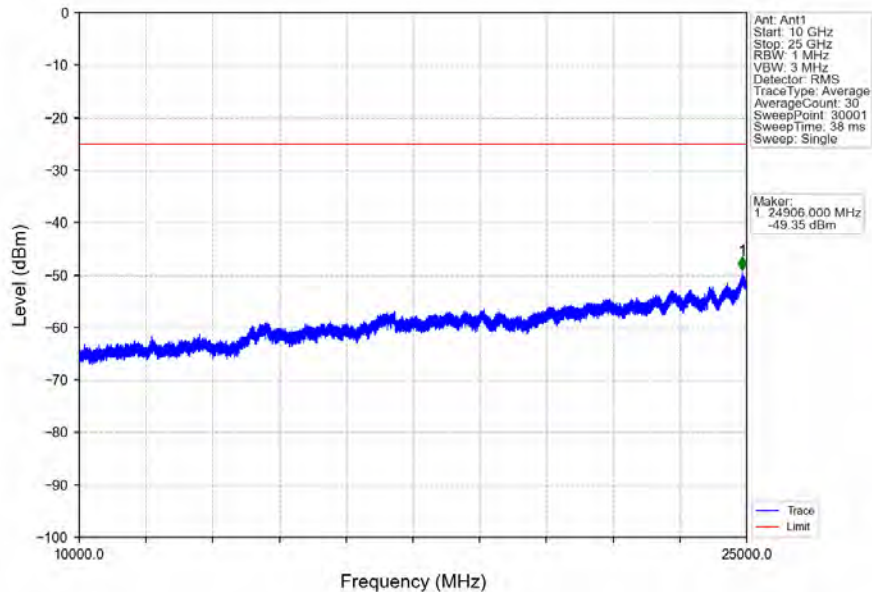
Band7_10MHz_QPSK_MCH_2535MHz_RB_1_0_NTNV
