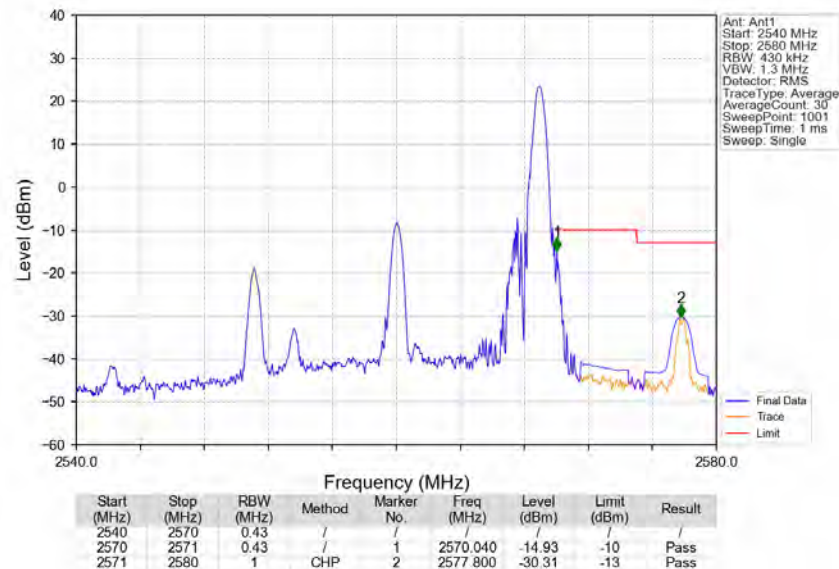
Band7_20MHz_QPSK_HCH_2560MHz_RB_1_99_NTNV
