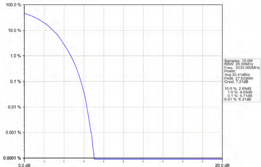
Band7_20MHz_64QAM_MCH_2535MHz_RB_100_0_NTNV
