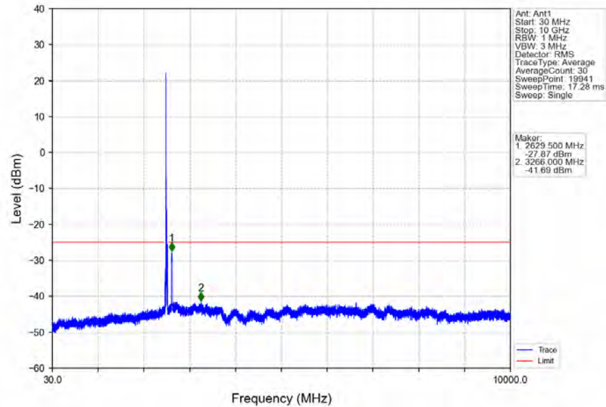
Band7_20MHz_16QAM_LCH_2510MHz_RB_1_0_NTNV
