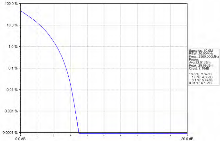
Band7_20MHz_QPSK_HCH_2560MHz_RB_100_0_NTNV
